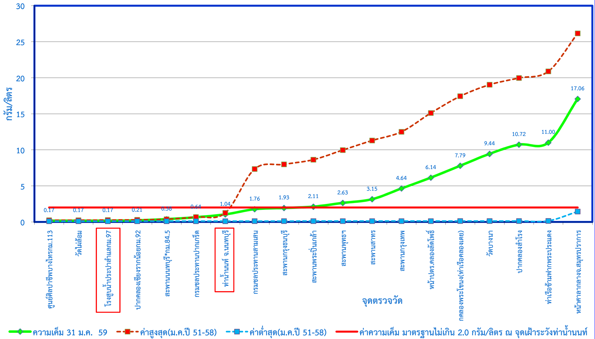
กราฟแสดงค่าความเค็มในแม่น้ำเจ้าพระยาตามพระราชเสาวนีย์ฯ เมื่อวันที่ 31 มกราคม 2559
