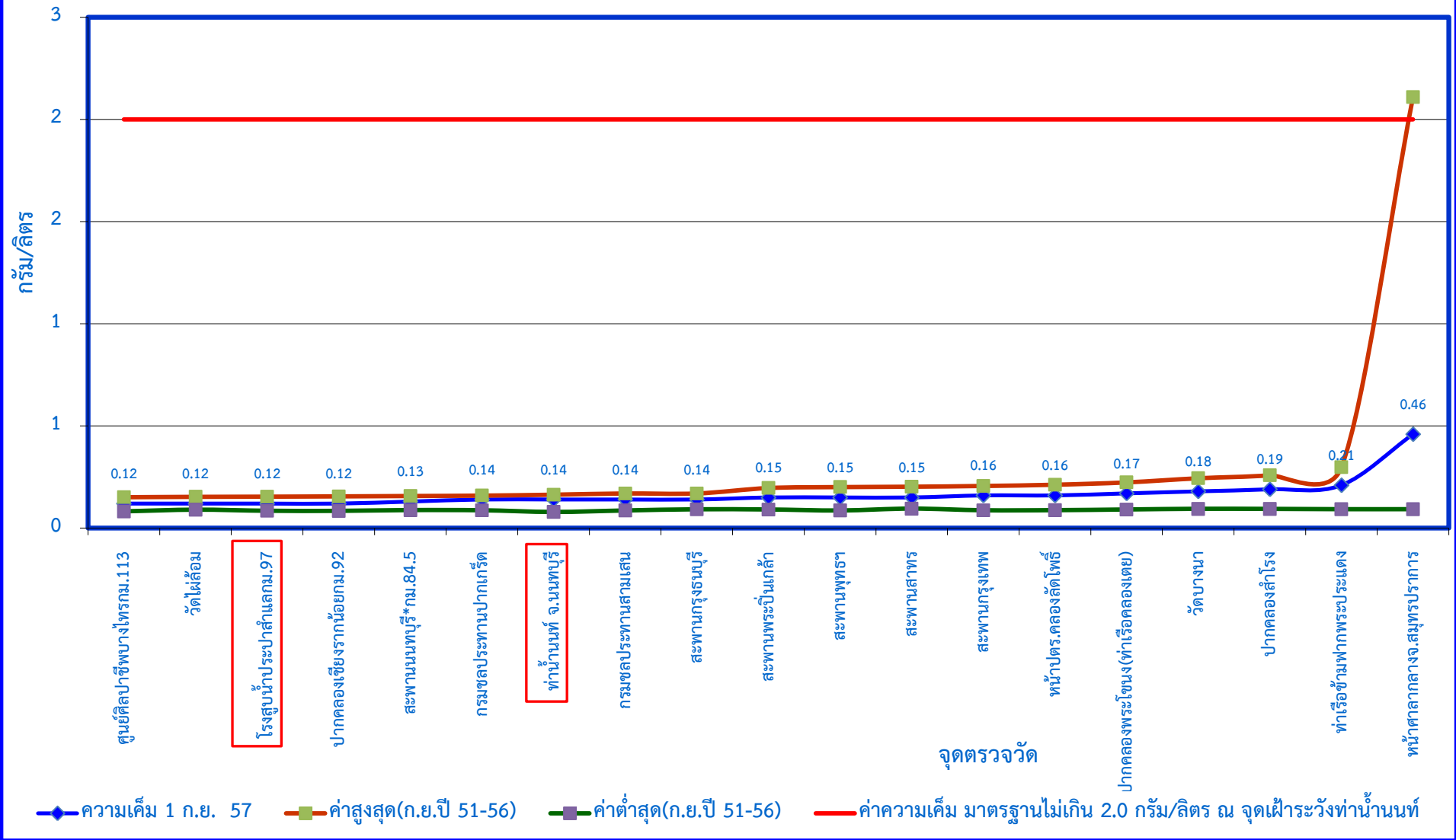
กราฟแสดงค่าความเค็มในแม่น้ำเจ้าพระยาตามพระราชเสาวนีย์ฯ เมื่อวันที่ 1 กันยายน 2557
