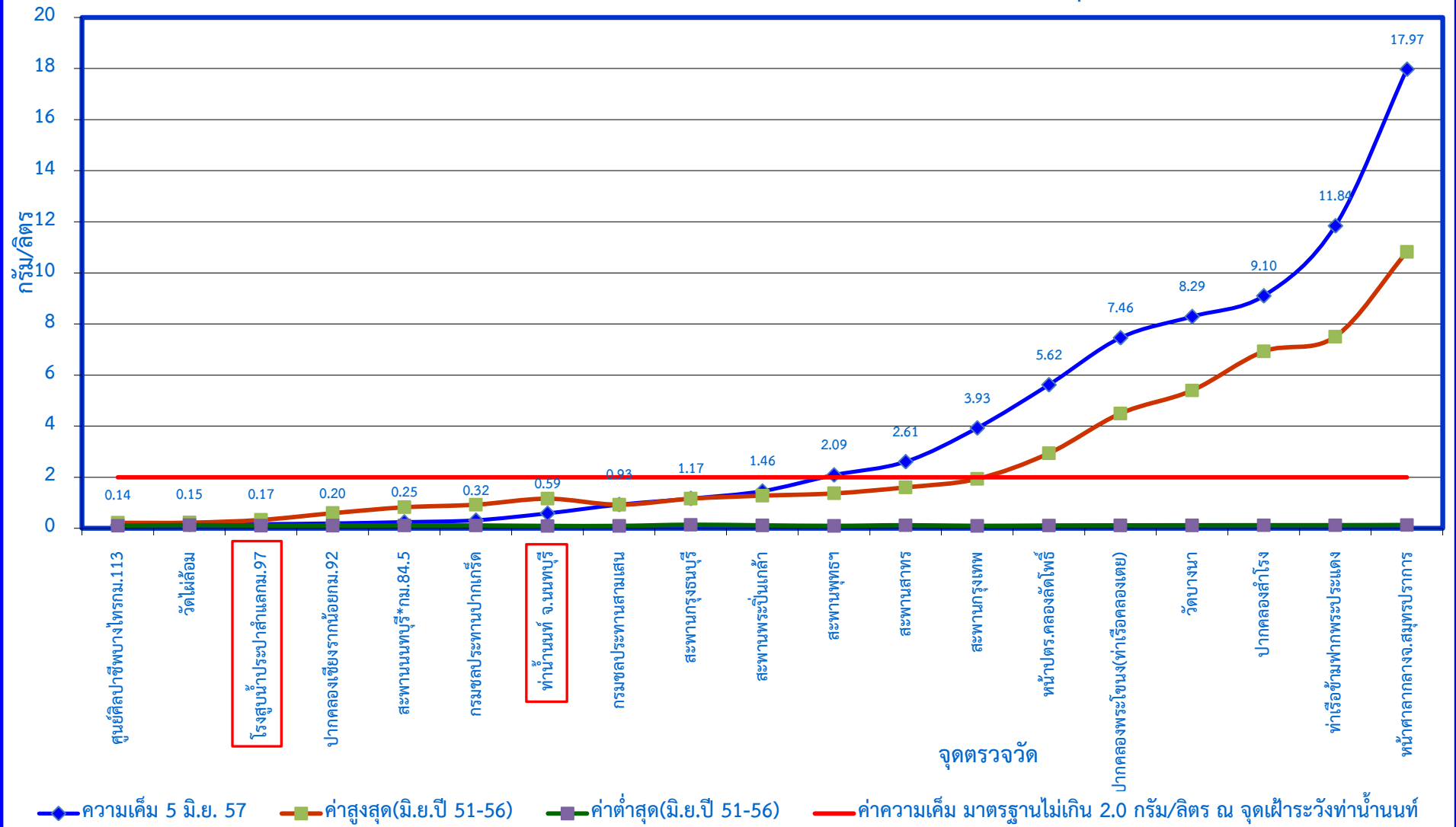
กราฟแสดงค่าความเค็มในแม่น้ำเจ้าพระยาตามพระราชเสาวนีย์ฯ เมื่อวันที่ 5 มิถุนายน 2557
