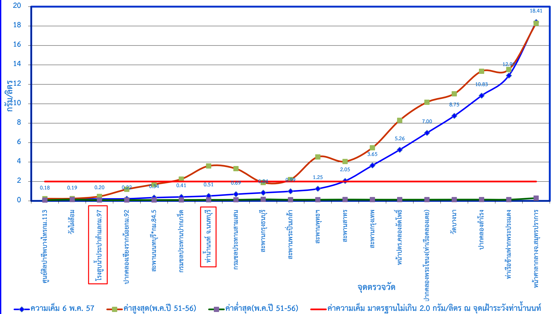
กราฟแสดงค่าความเค็มในแม่น้ำเจ้าพระยาตามพระราชเสาวนีย์ฯ เมื่อวันที่ 6 พฤษภาคม 2557
