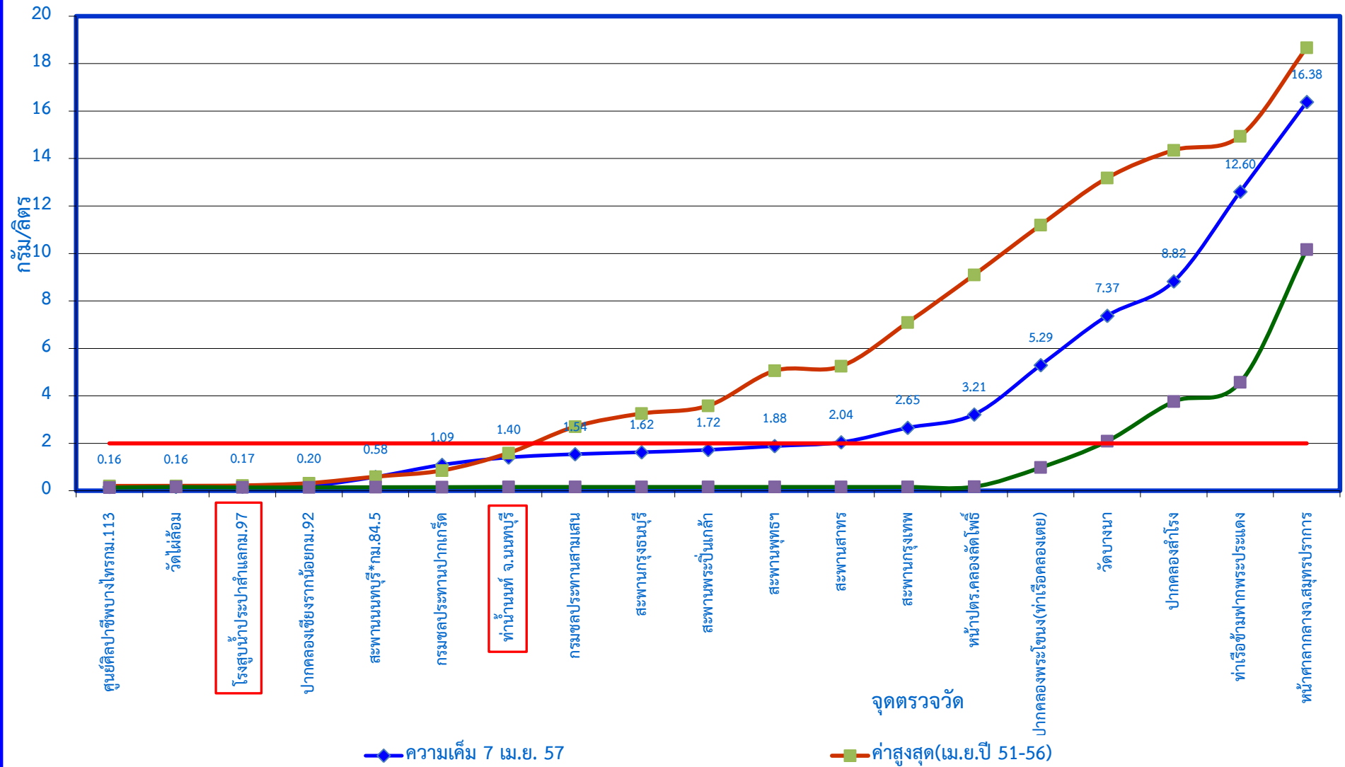
กราฟแสดงค่าความเค็มในแม่น้ำเจ้าพระยาตามพระราชเสาวนีย์ฯ เมื่อวันที่ 7 เมษายน 2557
