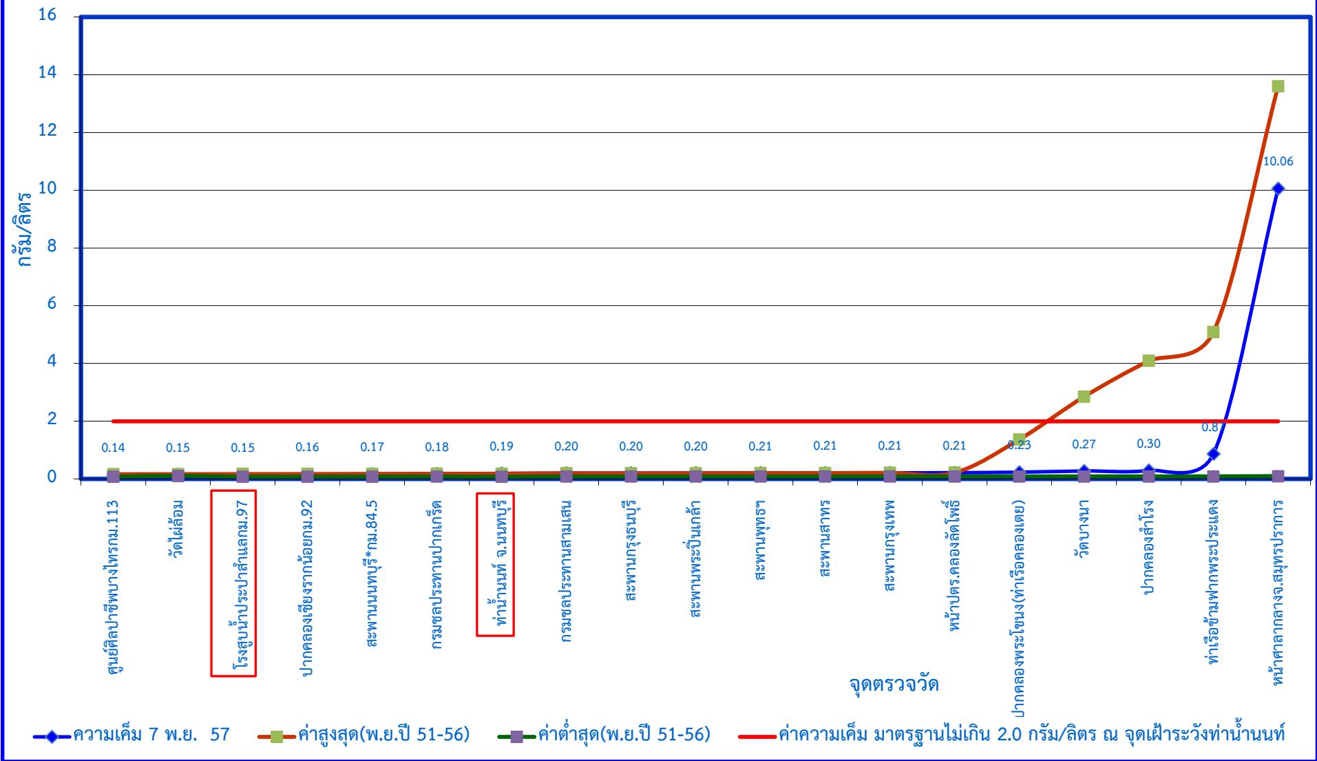
กราฟแสดงค่าความเค็มในแม่น้ำเจ้าพระยาตามพระราชเสาวนีย์ฯ เมื่อวันที่ 7 พฤศจิกายน 2557
