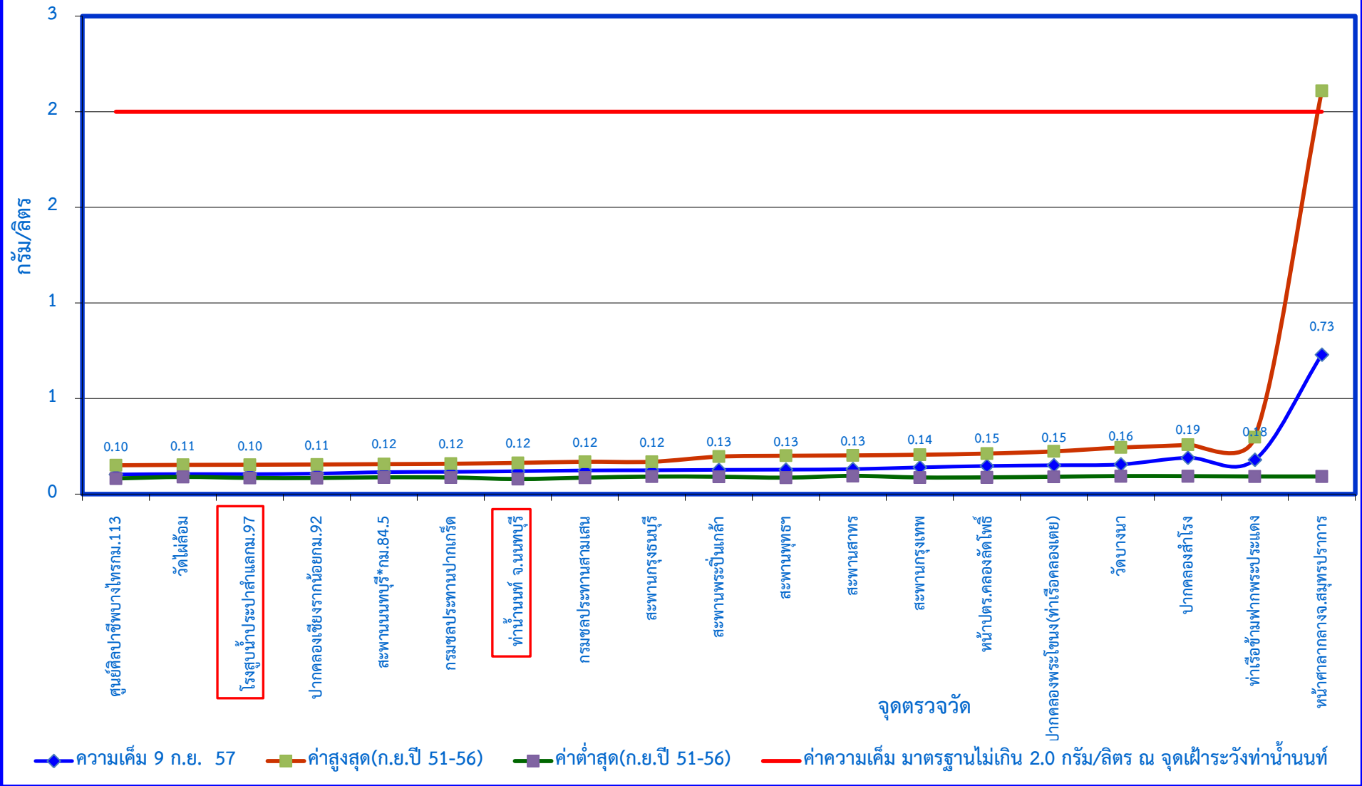
กราฟแสดงค่าความเค็มในแม่น้ำเจ้าพระยาตามพระราชเสาวนีย์ฯ เมื่อวันที่ 9 กันยายน 2557
