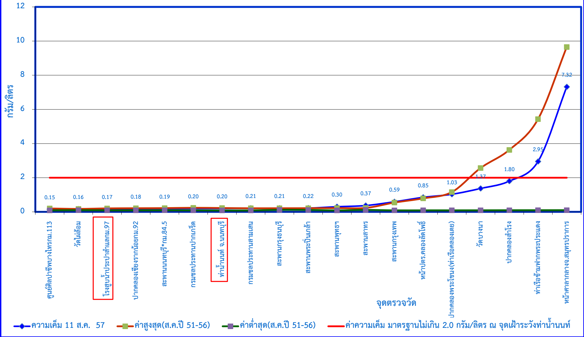
กราฟแสดงค่าความเค็มในแม่น้ำเจ้าพระยาตามพระราชเสาวนีย์ฯ เมื่อวันที่ 11 สิงหาคม 2557
