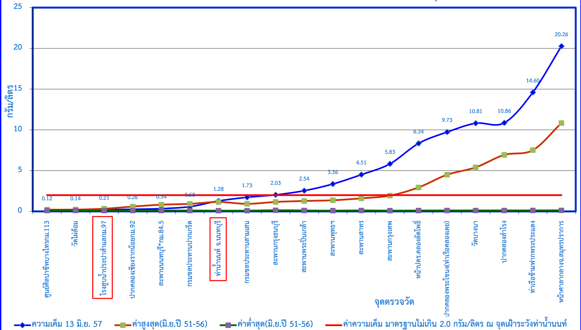
กราฟแสดงค่าความเค็มในแม่น้ำเจ้าพระยาตามพระราชเสาวนีย์ฯ เมื่อวันที่ 13 มิถุนายน 2557
