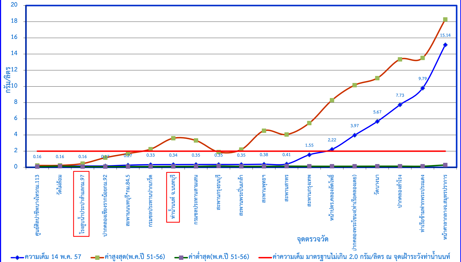
กราฟแสดงค่าความเค็มในแม่น้ำเจ้าพระยาตามพระราชเสาวนีย์ฯ เมื่อวันที่ 14 พฤษภาคม 2557
