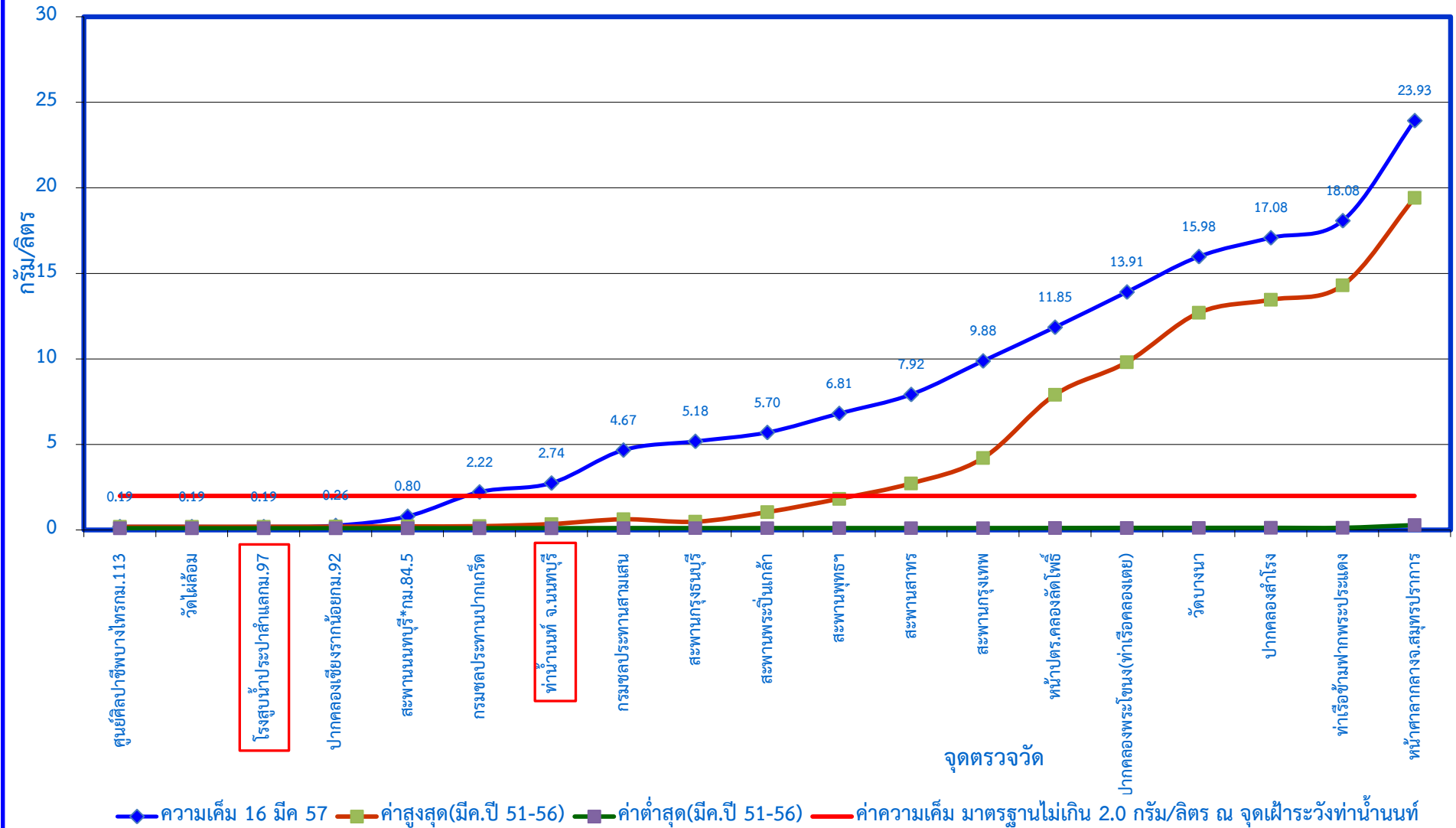
กราฟแสดงค่าความเค็มในแม่น้ำเจ้าพระยาตามพระราชเสาวนีย์ฯ เมื่อวันที่ ๑๖ มีนาคม ๒๕๕๗
