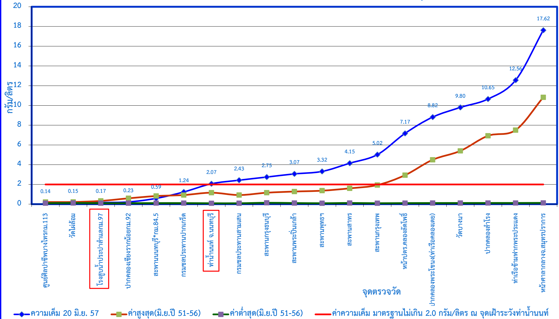
กราฟแสดงค่าความเค็มในแม่น้ำเจ้าพระยาตามพระราชเสาวนีย์ฯ เมื่อวันที่ 20 มิถุนายน 2557
