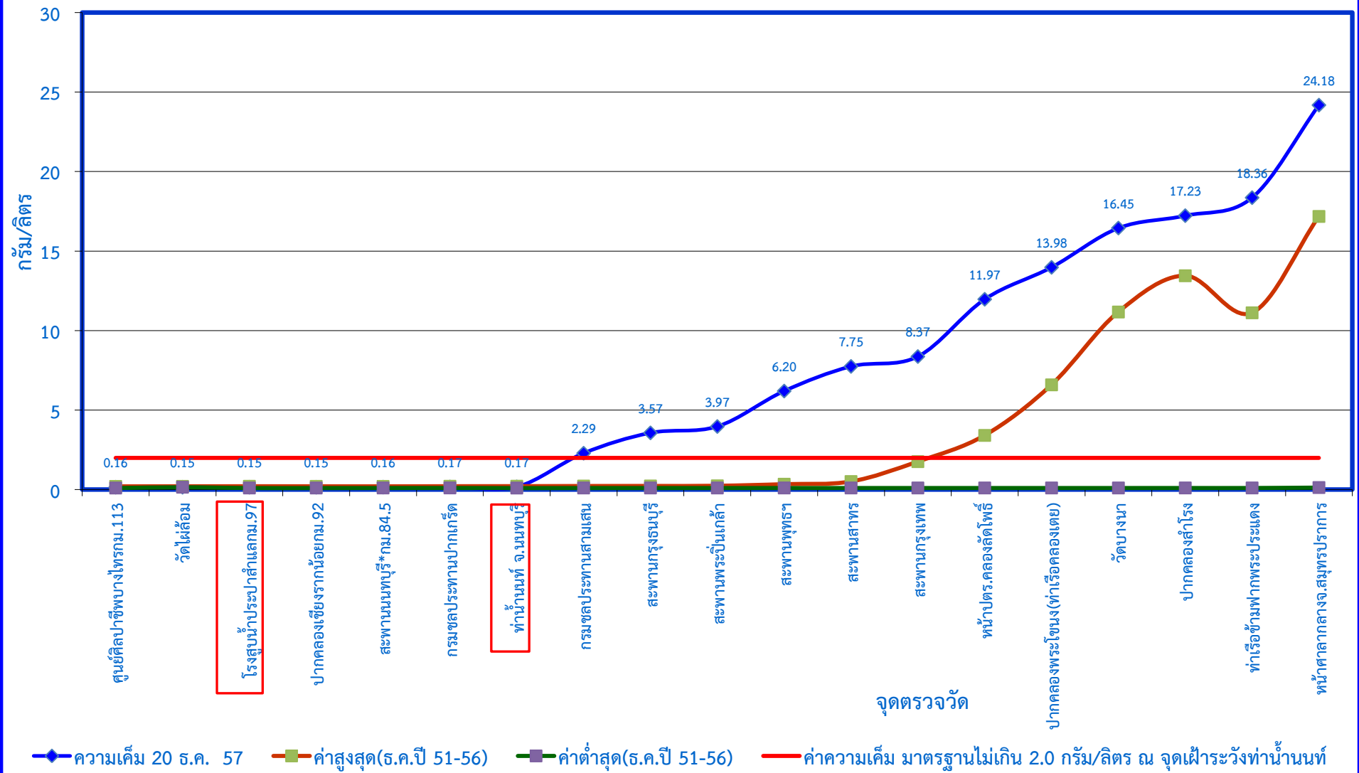
กราฟแสดงค่าความเค็มในแม่น้ำเจ้าพระยาตามพระราชเสาวนีย์ฯ เมื่อวันที่ 20 ธันวาคม 2557
