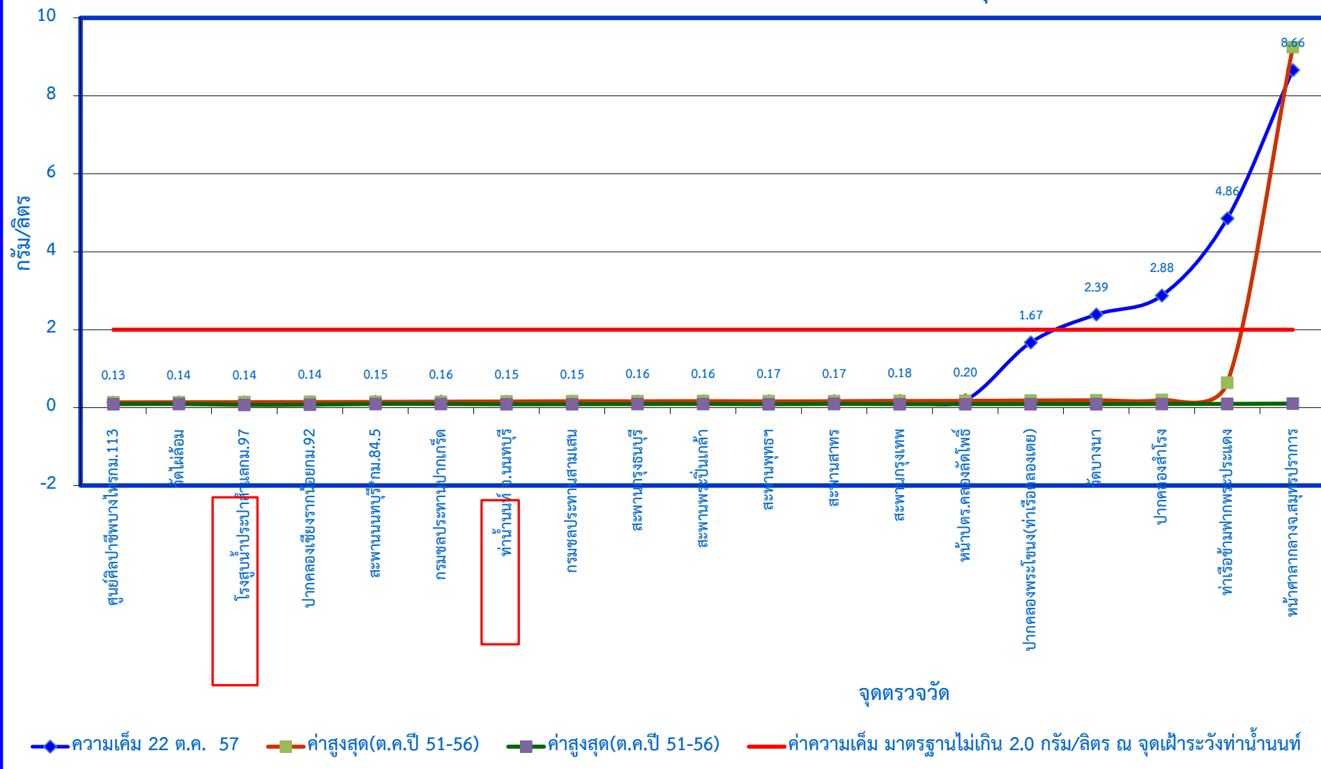
กราฟแสดงค่าความเค็มในแม่น้ำเจ้าพระยาตามพระราชเสาวนีย์ฯ เมื่อวันที่ 22 ตุลาคม 2557
