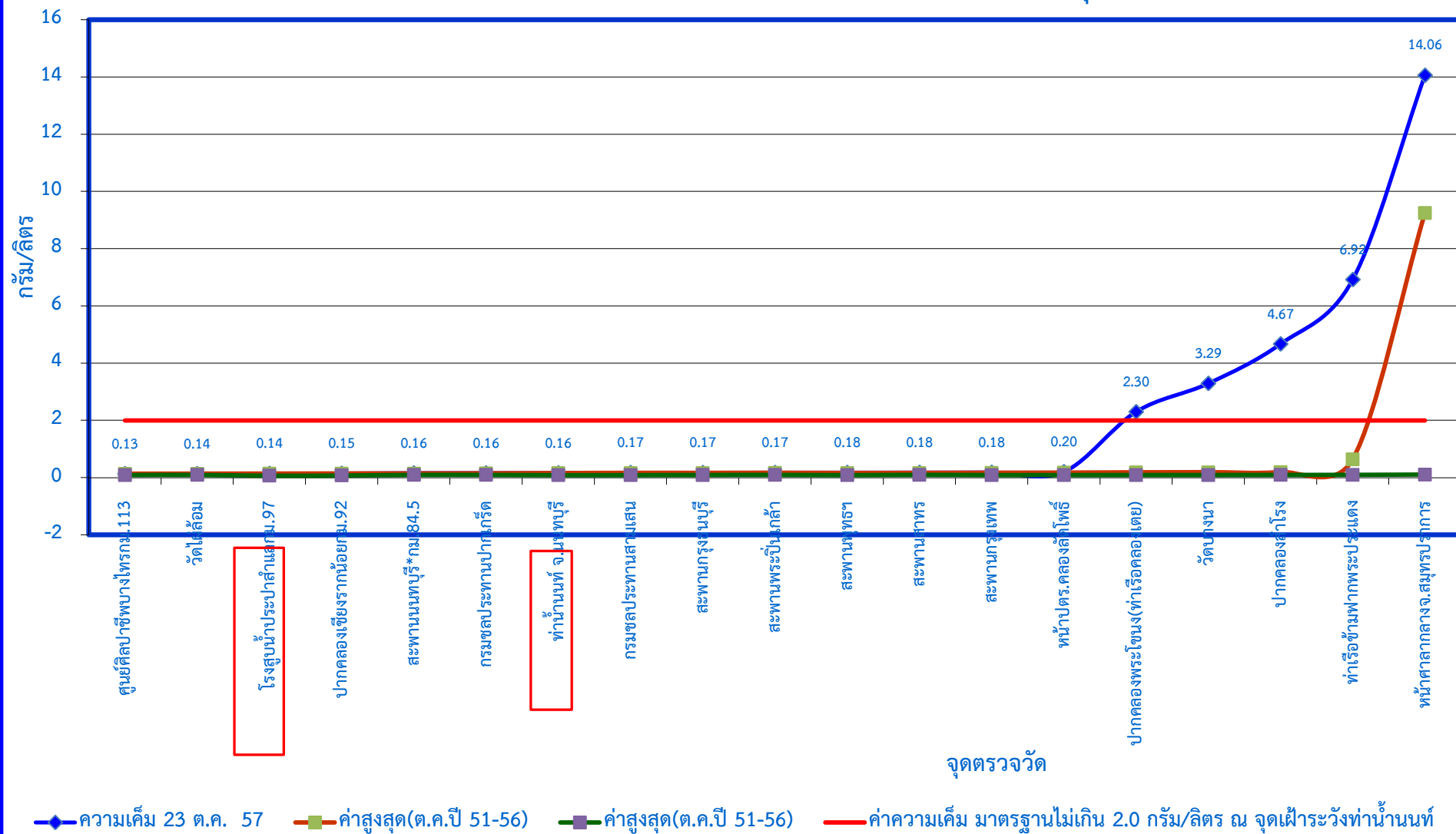
กราฟแสดงค่าความเค็มในแม่น้ำเจ้าพระยาตามพระราชเสาวนีย์ฯ เมื่อวันที่ 23 ตุลาคม 2557
