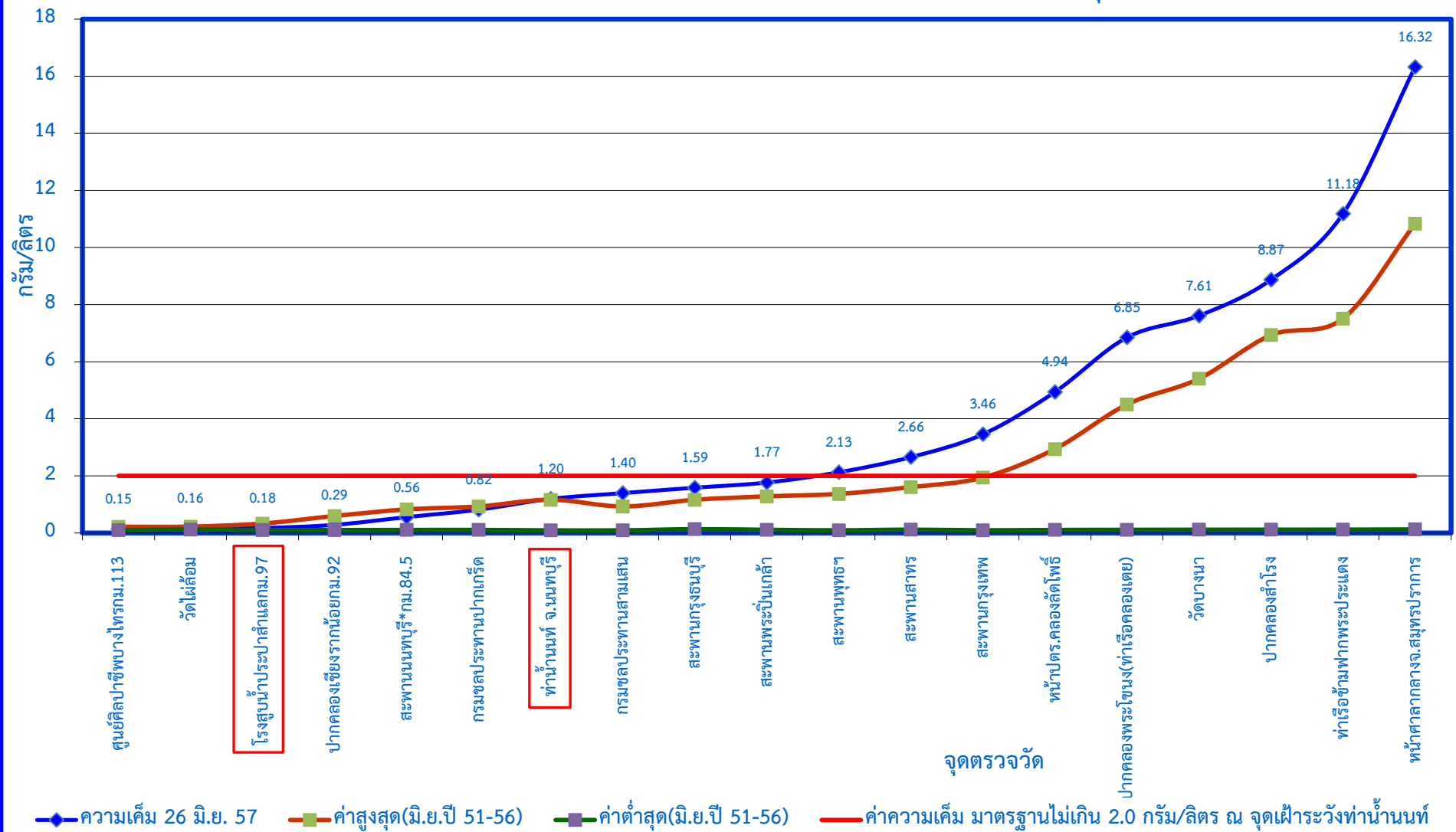
กราฟแสดงค่าความเค็มในแม่น้ำเจ้าพระยาตามพระราชเสาวนีย์ฯ เมื่อวันที่ 26 มิถุนายน 2557
