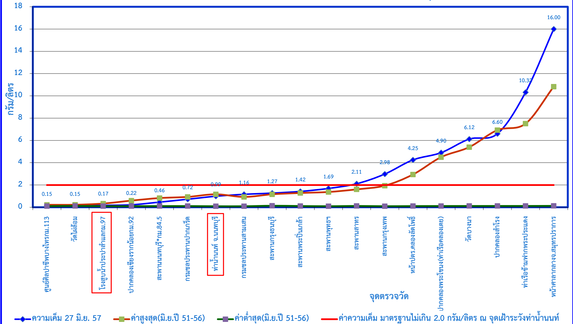
กราฟแสดงค่าความเค็มในแม่น้ำเจ้าพระยาตามพระราชเสาวนีย์ฯ เมื่อวันที่ 27 มิถุนายน 2557
