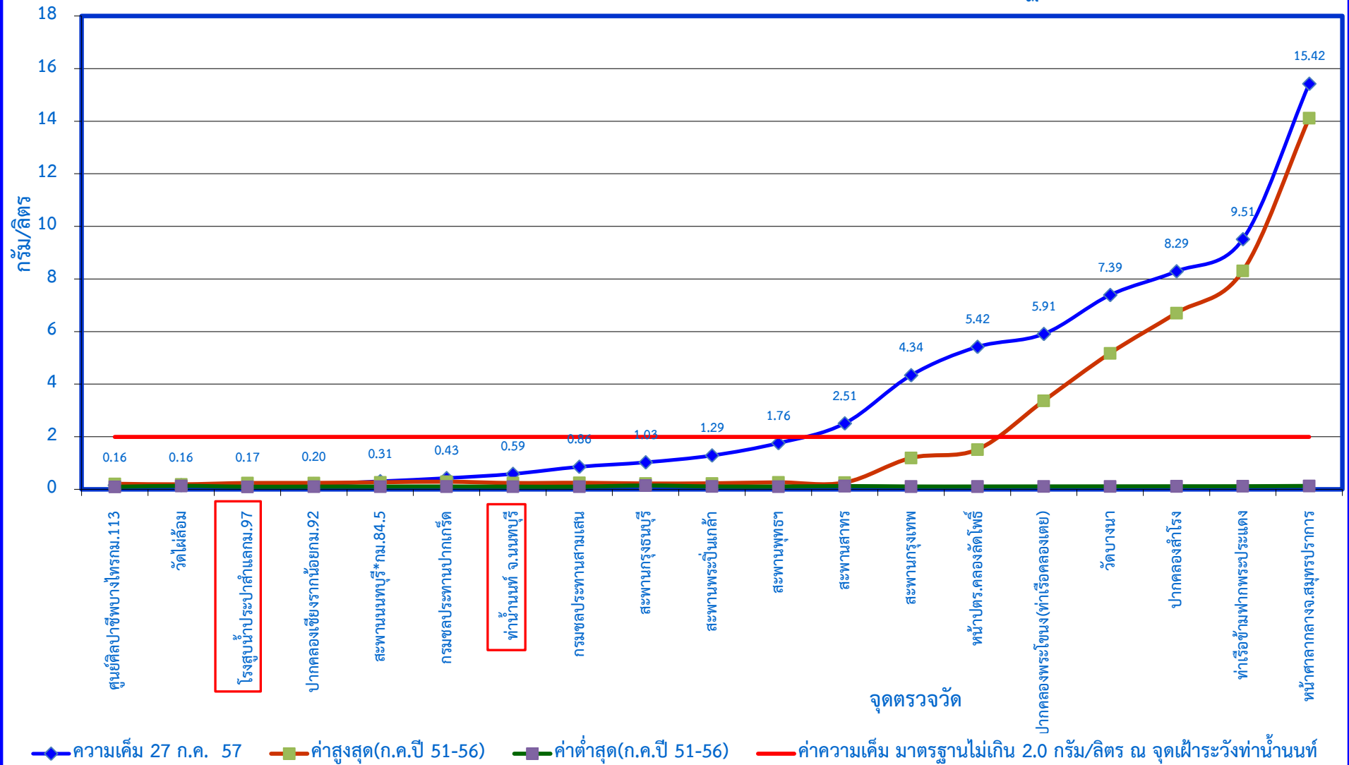
กราฟแสดงค่าความเค็มในแม่น้ำเจ้าพระยาตามพระราชเสาวนีย์ฯ เมื่อวันที่ 27 กรกฎาคม 2557
