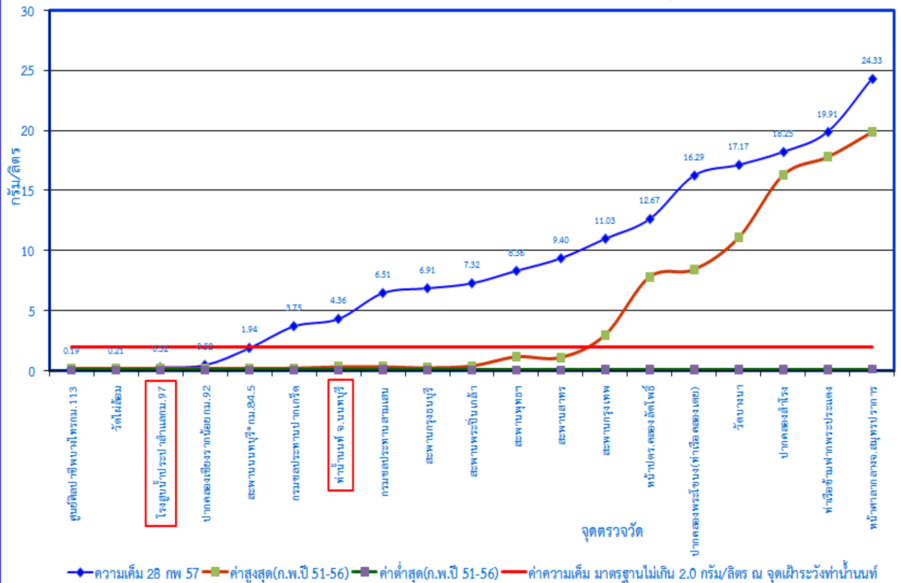
กราฟแสดงค่าความเค็มในแม่น้ำเจ้าพระยาตามพระราชเสาวนีย์ฯ เมื่อวันที่ ๒๘ กุมภาพันธ์ ๒๕๕๗
