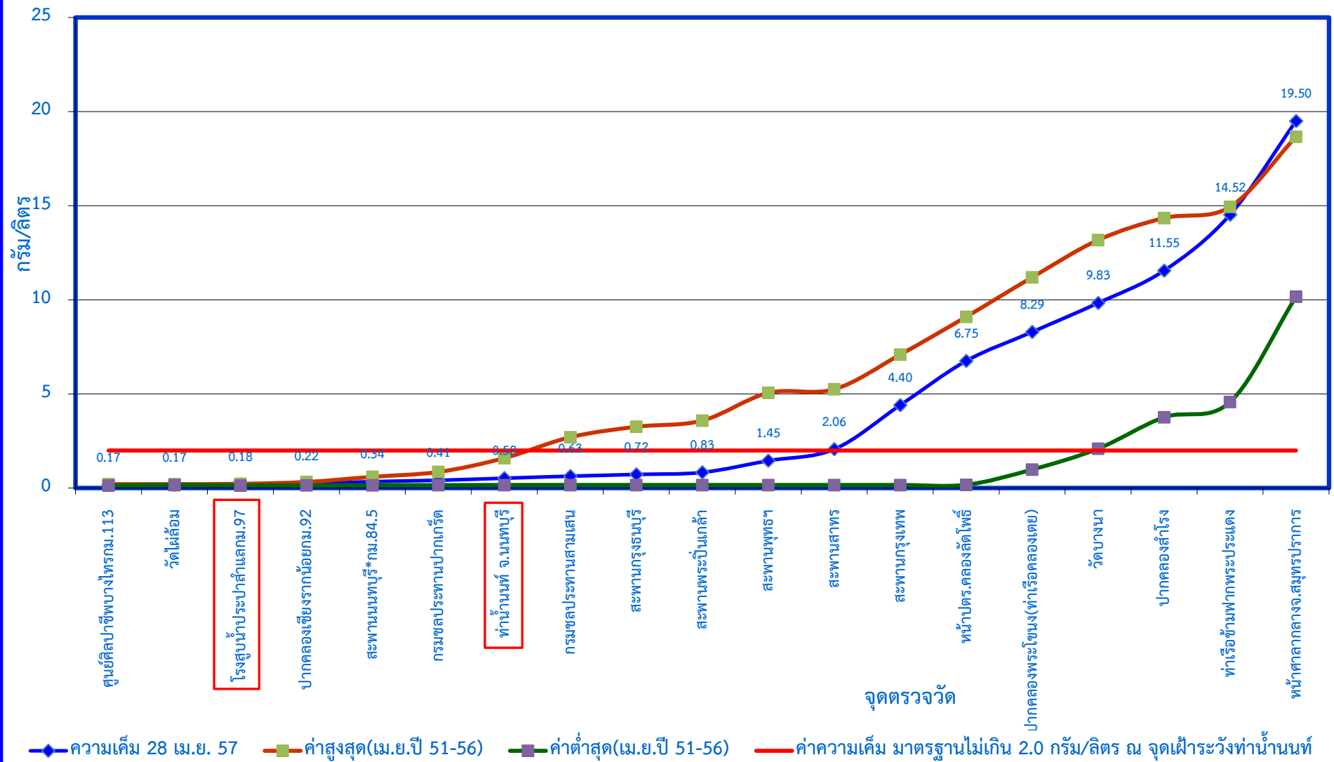
กราฟแสดงค่าความเค็มในแม่น้ำเจ้าพระยาตามพระราชเสาวนีย์ฯ เมื่อวันที่ 28 เมษายน 2557
