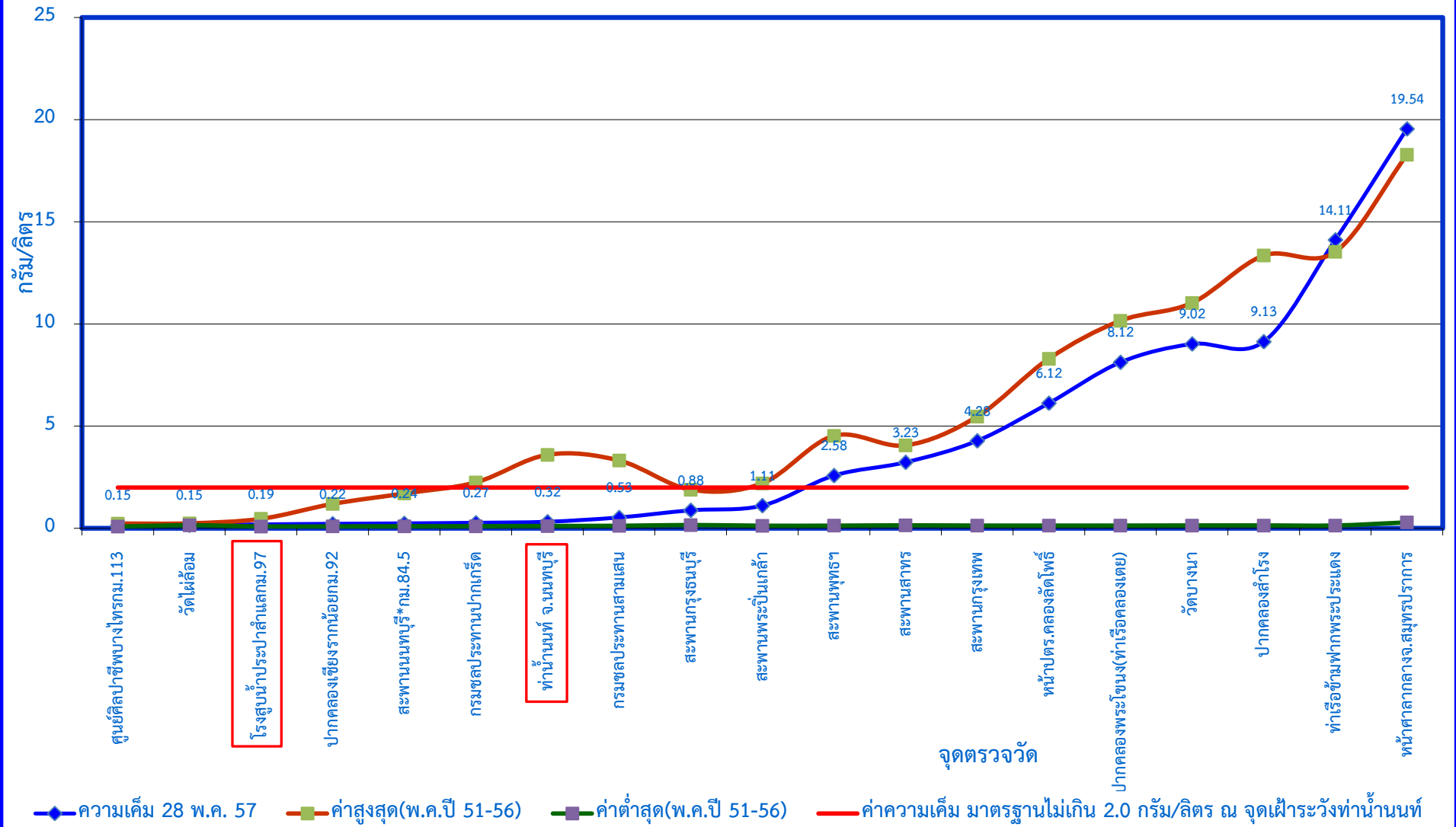
กราฟแสดงค่าความเค็มในแม่น้ำเจ้าพระยาตามพระราชเสาวนีย์ฯ เมื่อวันที่ 28 พฤษภาคม 2557
