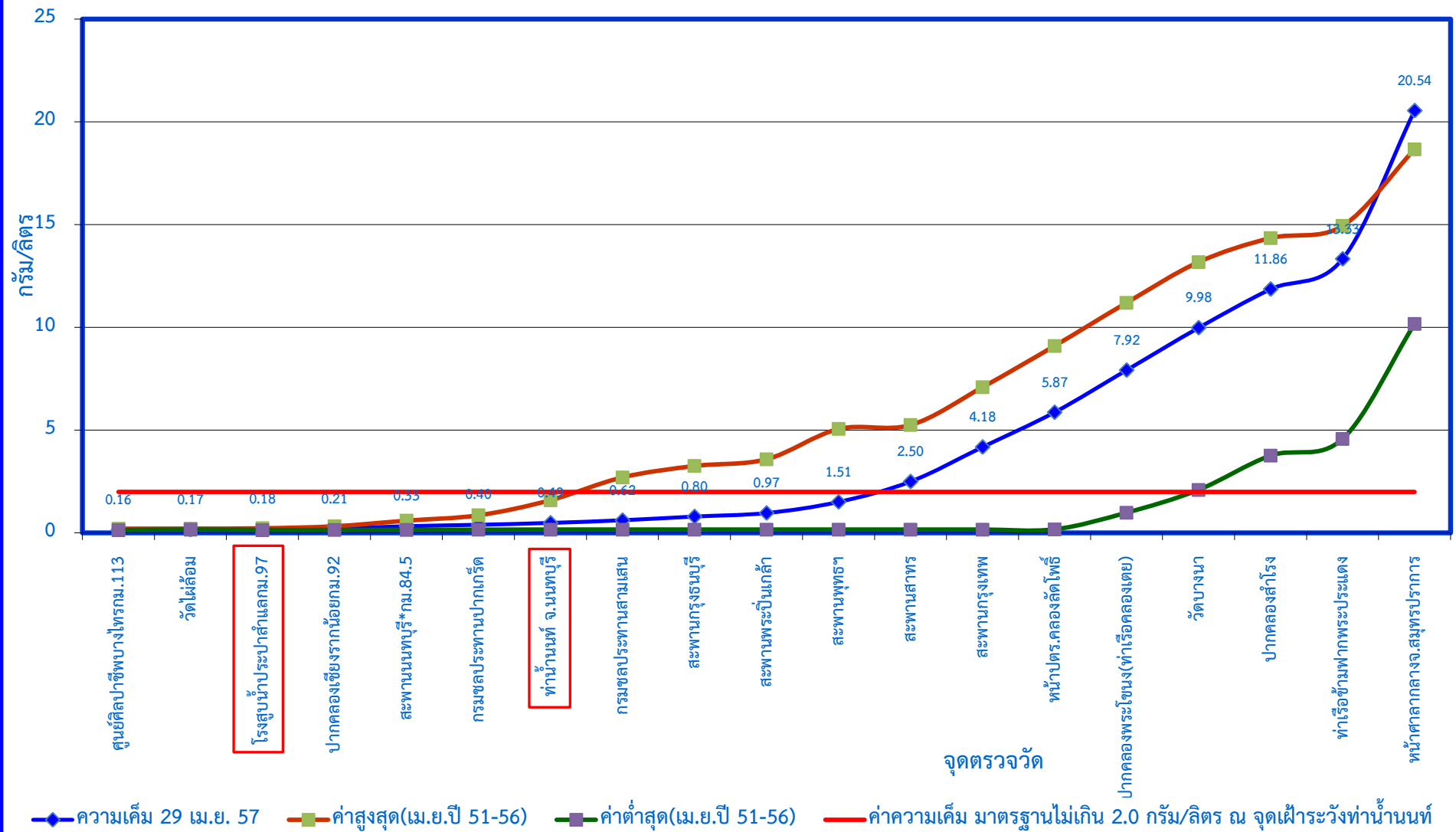
กราฟแสดงค่าความเค็มในแม่น้ำเจ้าพระยาตามพระราชเสาวนีย์ฯ เมื่อวันที่ 29 เมษายน 2557
