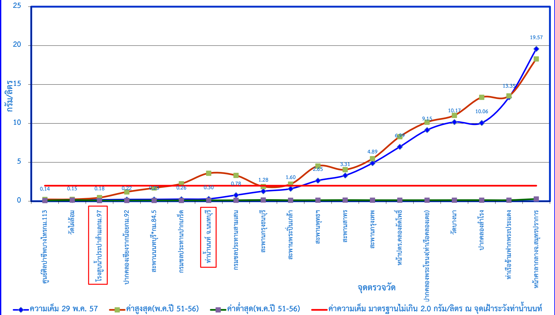
กราฟแสดงค่าความเค็มในแม่น้ำเจ้าพระยาตามพระราชเสาวนีย์ฯ เมื่อวันที่ 29 พฤษภาคม 2557
