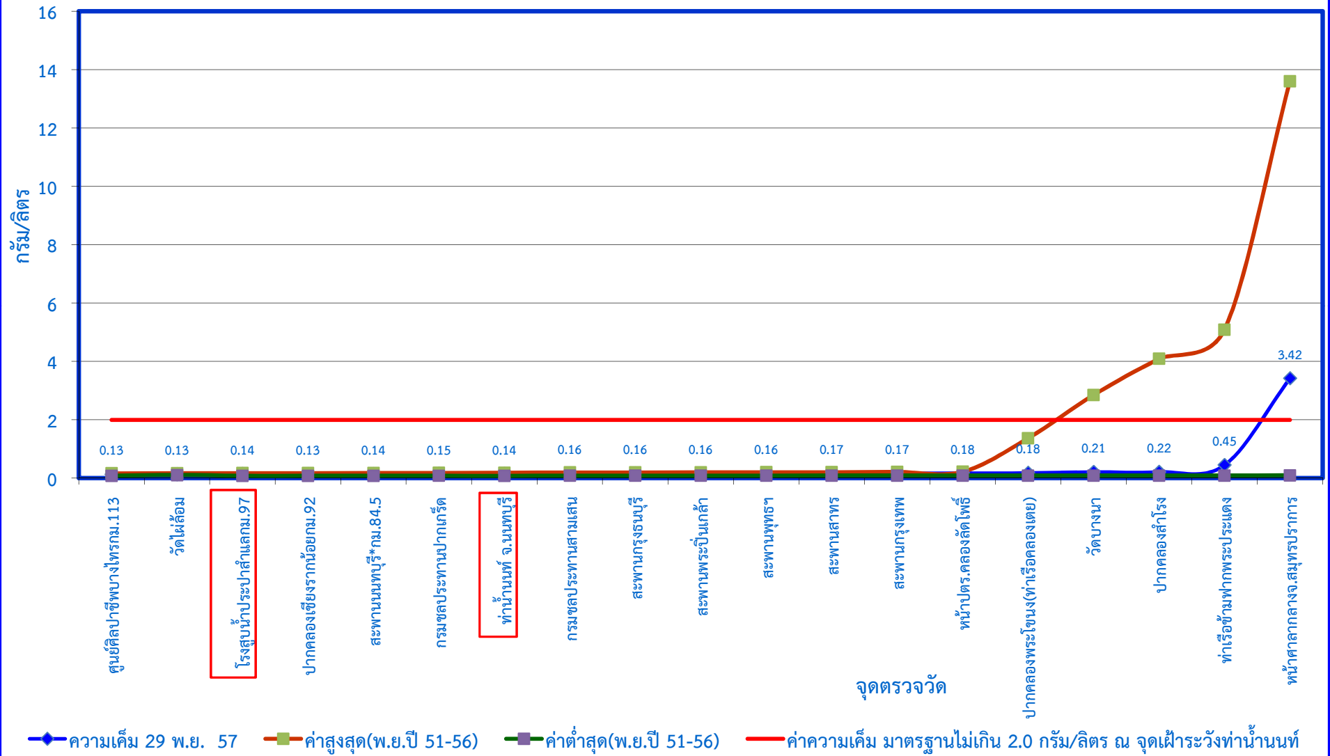
กราฟแสดงค่าความเค็มในแม่น้ำเจ้าพระยาตามพระราชเสาวนีย์ฯ เมื่อวันที่ 29 พฤศจิกายน 2557
