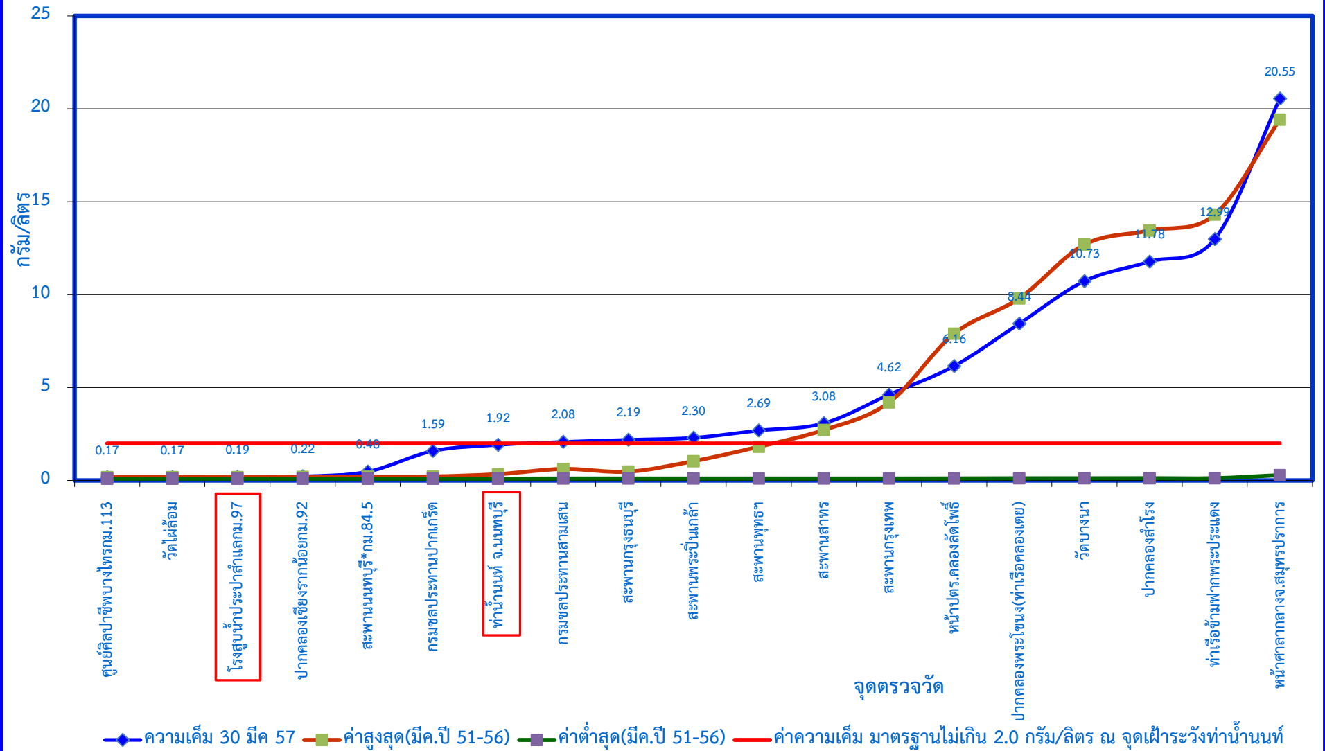
กราฟแสดงค่าความเค็มในแม่น้ำเจ้าพระยาตามพระราชเสาวนีย์ฯ เมื่อวันที่ 30 มีนาคม 2557
