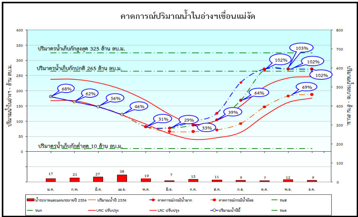
รูปที่ 3 การคาดการณ์ปริมาณน้ำเขื่อนแม่งัด กรณีปีน้ำเฉลี่ย ของปี พ.ศ. 2556
