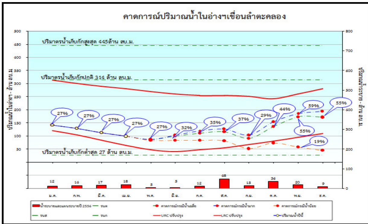
รูปที่ 14 การคาดการณ์ปริมาณน้ำเขื่อนลำตะคอง กรณีปีน้ำเฉลี่ย ของปี พ.ศ. 2556
