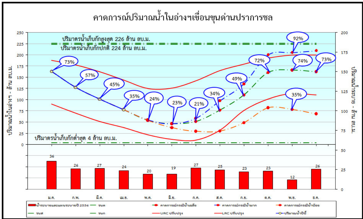
รูปที่ 25 การคาดการณ์ปริมาณน้ำเขื่อนขุนด่านปราการชล กรณีปีน้ำเฉลี่ย ของปี พ.ศ. 2556
