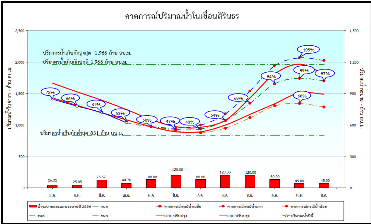
รูปที่ 19 การคาดการณ์ปริมาณน้ำเขื่อนสิรินธร กรณีปีน้ำเฉลี่ย ของปี พ.ศ. 2556
