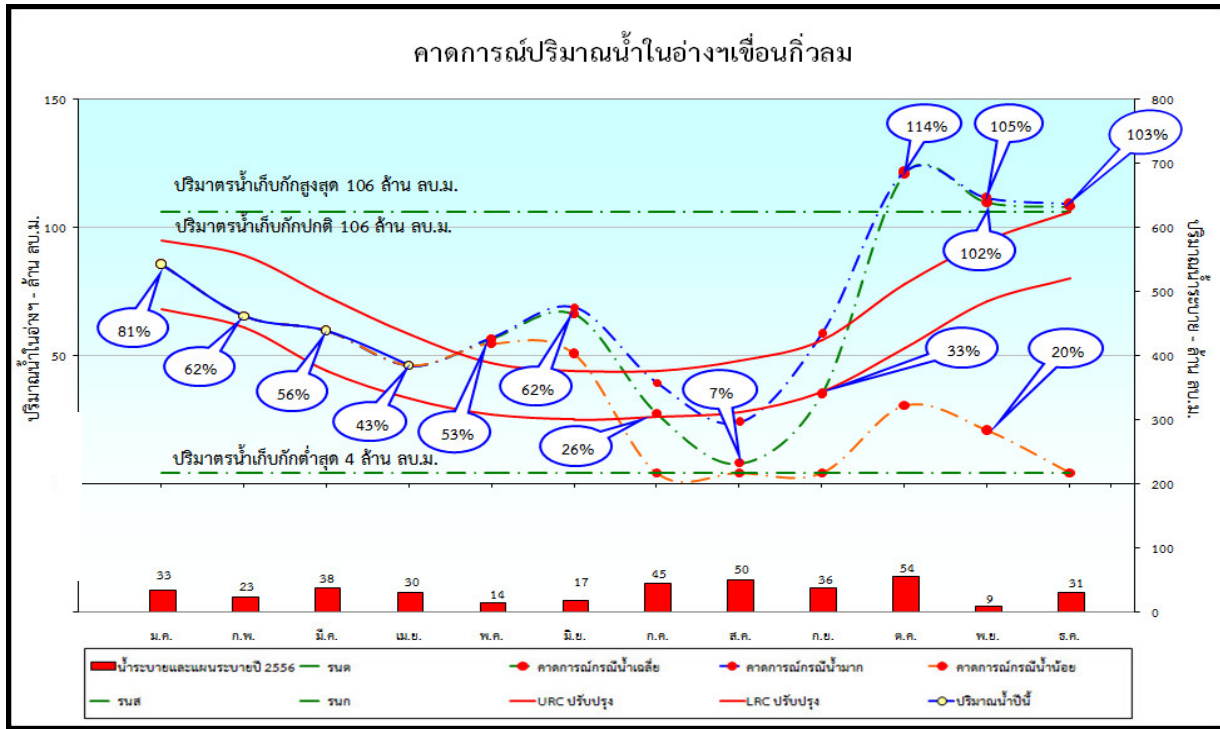
รูปที่ 5 การคาดการณ์ปริมาณน้ำเขื่อนกิ่วลม กรณีปีน้ำเฉลี่ย ของปี พ.ศ. 2556
