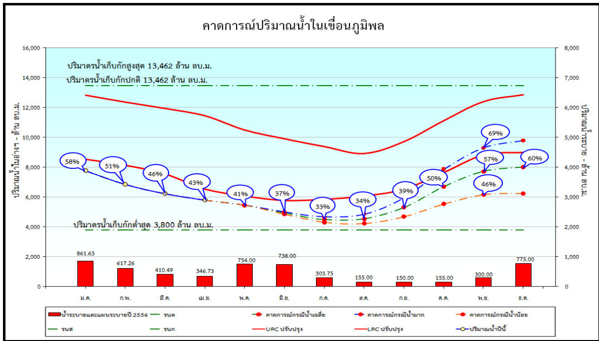
รูปที่ 1 การคาดการณ์ปริมาณน้ำเขื่อนภูมิพล กรณีปีน้ำเฉลี่ย ของปี พ.ศ. 2556
