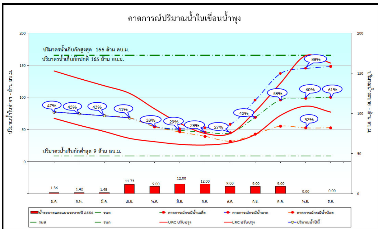
รูปที่ 10 การคาดการณ์ปริมาณน้ำเขื่อนน้ำพุง กรณีปีน้ำเฉลี่ย ของปี พ.ศ. 2556
