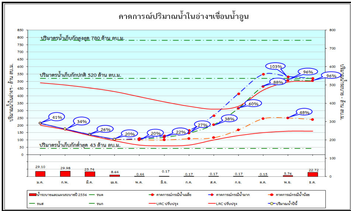
รูปที่ 9 การคาดการณ์ปริมาณน้ำเขื่อนน้ำอูน กรณีปีน้ำเฉลี่ย ของปี พ.ศ. 2556
