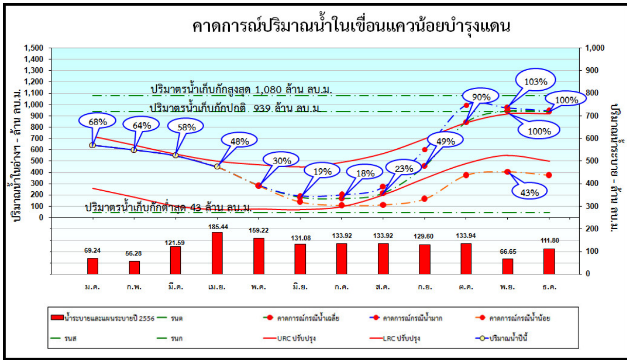
รูปที่ 7 การคาดการณ์ปริมาณน้ำเขื่อนแควน้อยบำรุงแดน กรณีปีน้ำเฉลี่ย ของปี พ.ศ. 2556
