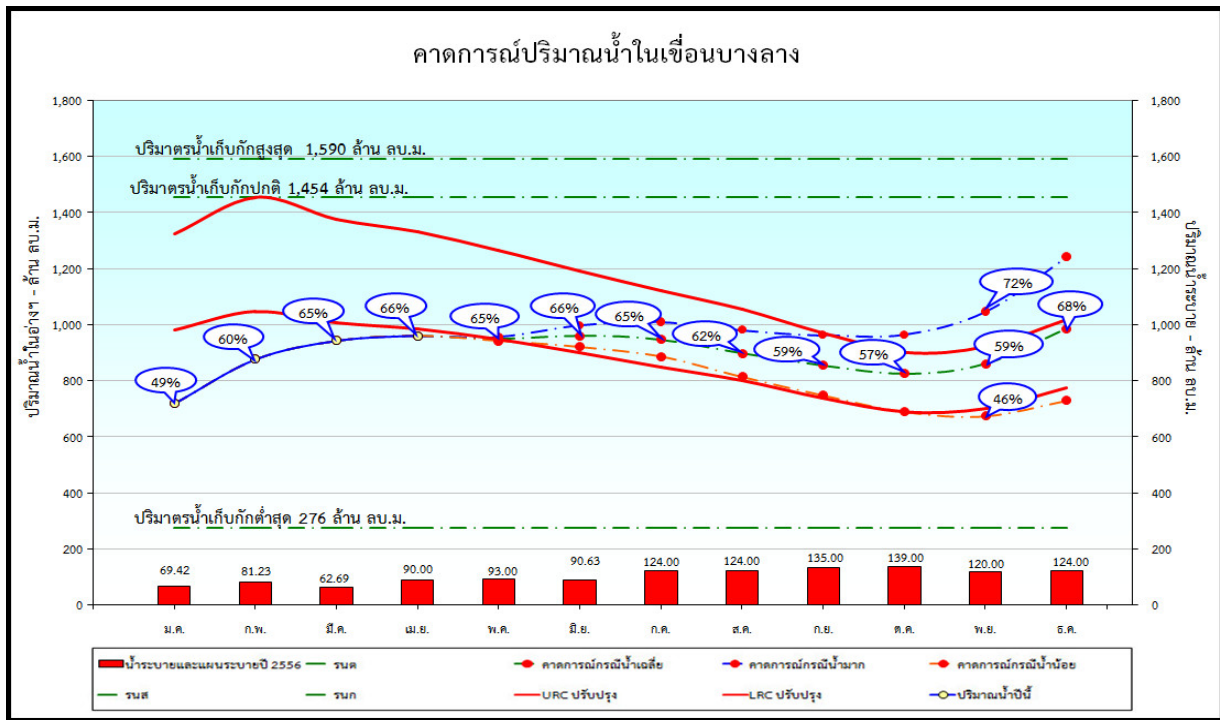
รูปที่ 33 การคาดการณ์ปริมาณน้ำเขื่อนบางลาง กรณีปีน้ำเฉลี่ย ของปี พ.ศ. 2556
