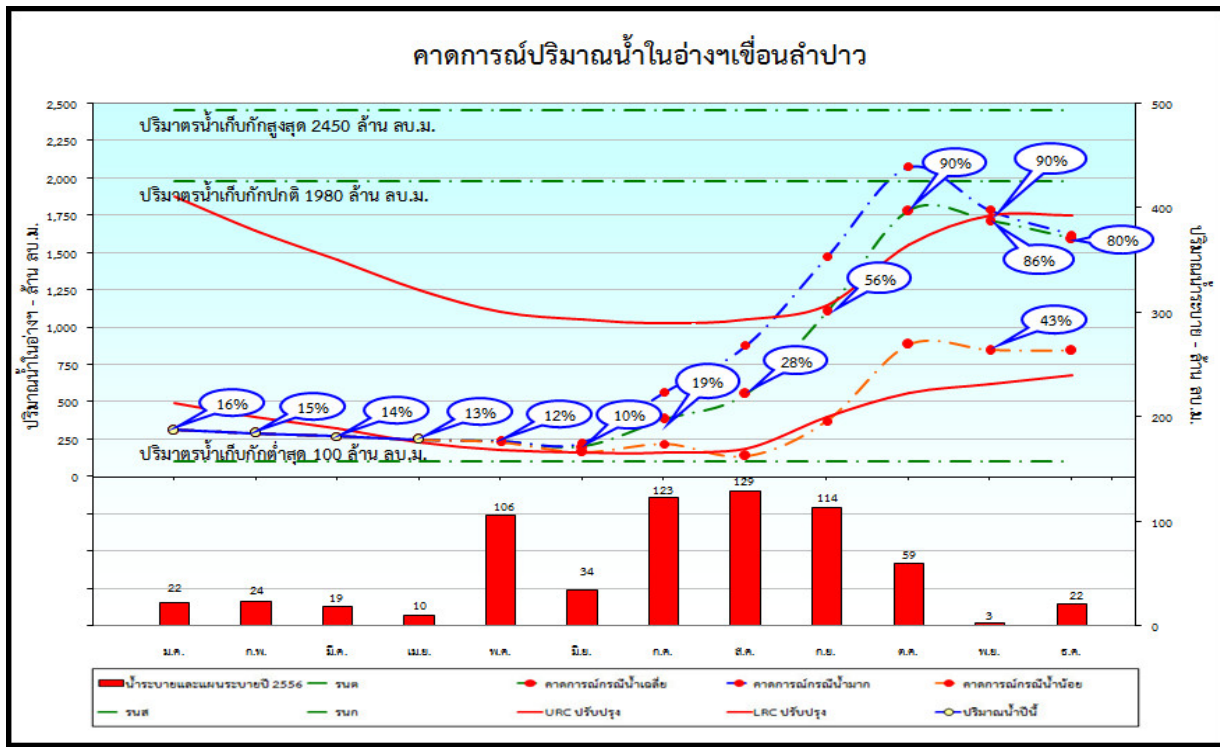
รูปที่ 13 การคาดการณ์ปริมาณน้ำเขื่อนลำปาว กรณีปีน้ำเฉลี่ย ของปี พ.ศ. 2556
