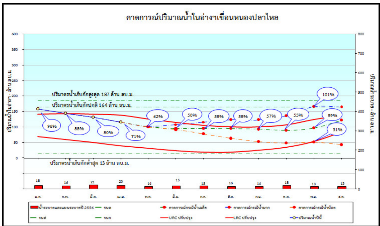
รูปที่ 28 การคาดการณ์ปริมาณน้ำเขื่อนหนองปลาไหล กรณีปีน้ำเฉลี่ย ของปี พ.ศ. 2556
