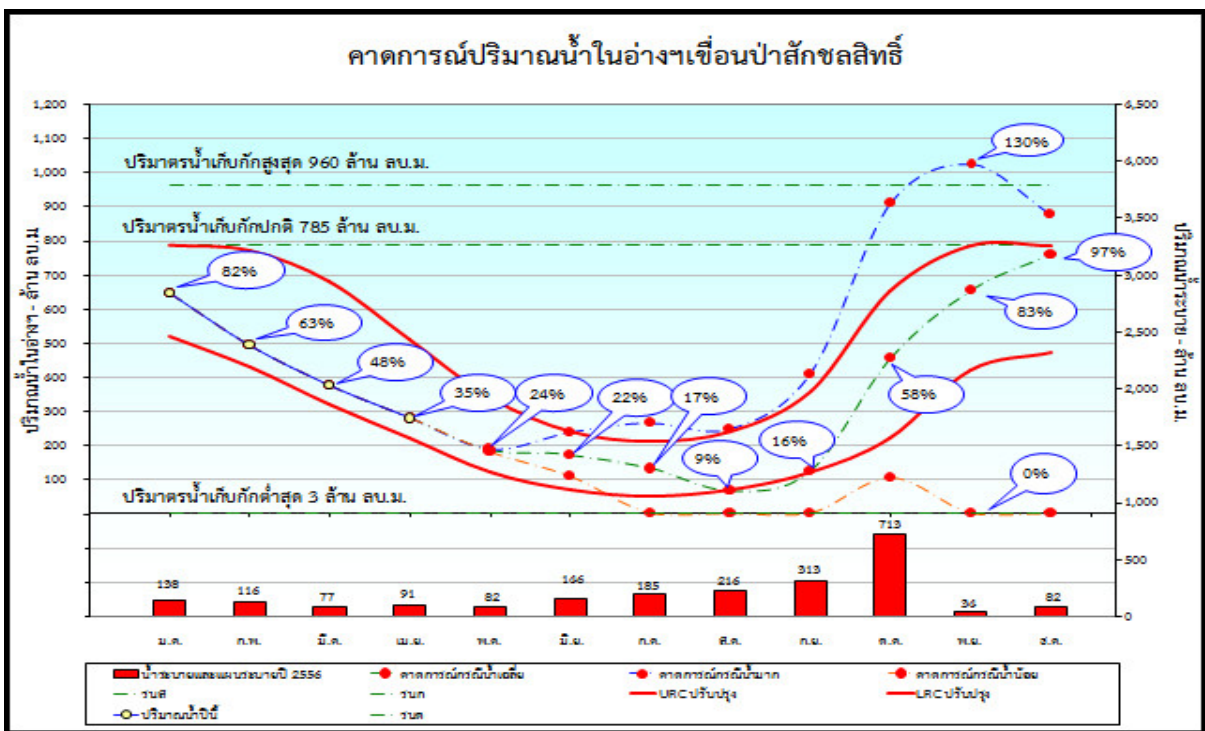
รูปที่ 20 การคาดการณ์ปริมาณน้ำเขื่อนป่าสักชลสิทธิ์ กรณีปีน้ำเฉลี่ย ของปี พ.ศ. 2556
