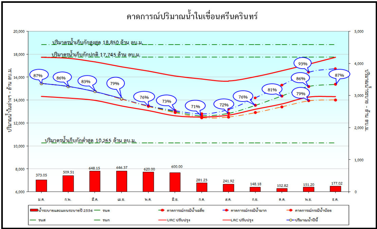
รูปที่ 23 การคาดการณ์ปริมาณน้ำเขื่อนศรีนครินทร์ กรณีปีน้ำเฉลี่ย ของปี พ.ศ. 2556
