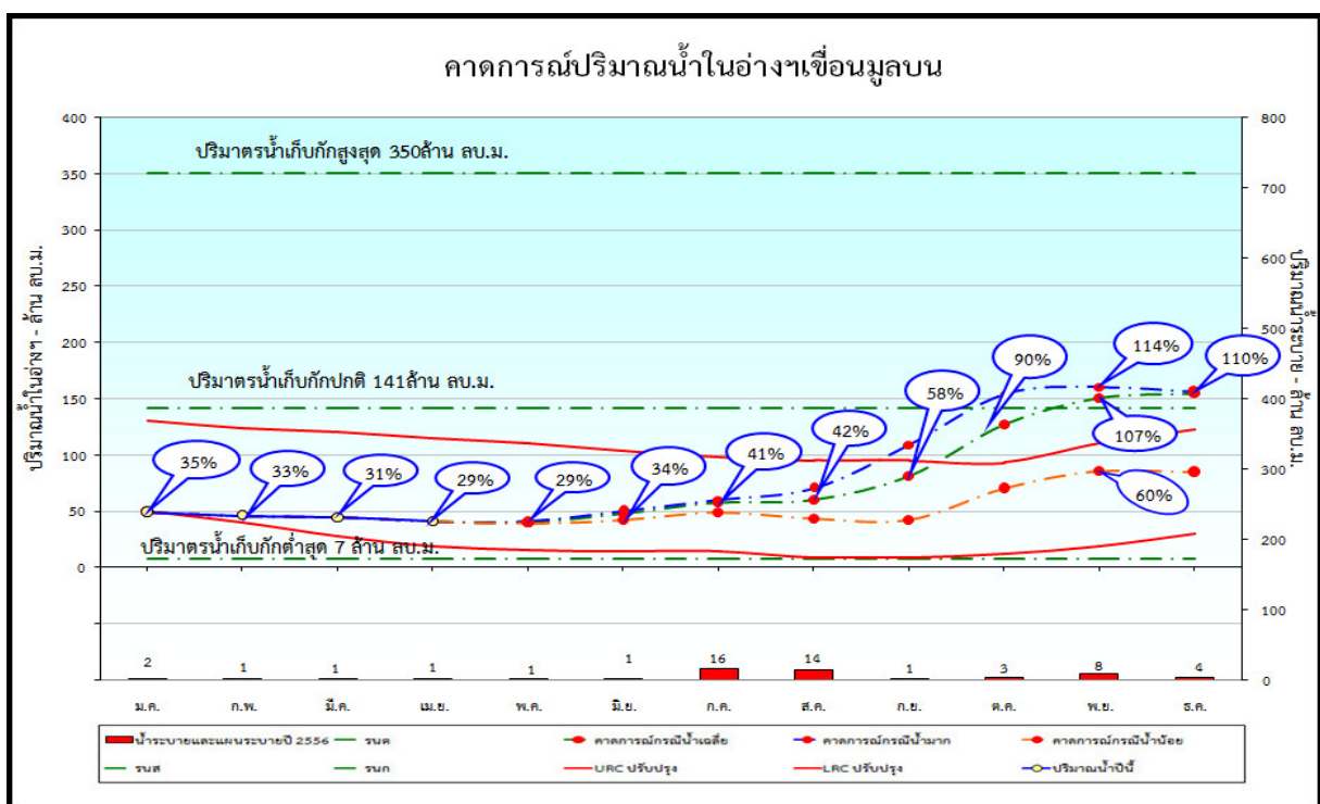
รูปที่ 16 การคาดการณ์ปริมาณน้ำเขื่อนมูลบน กรณีปีน้ำเฉลี่ย ของปี พ.ศ. 2556
