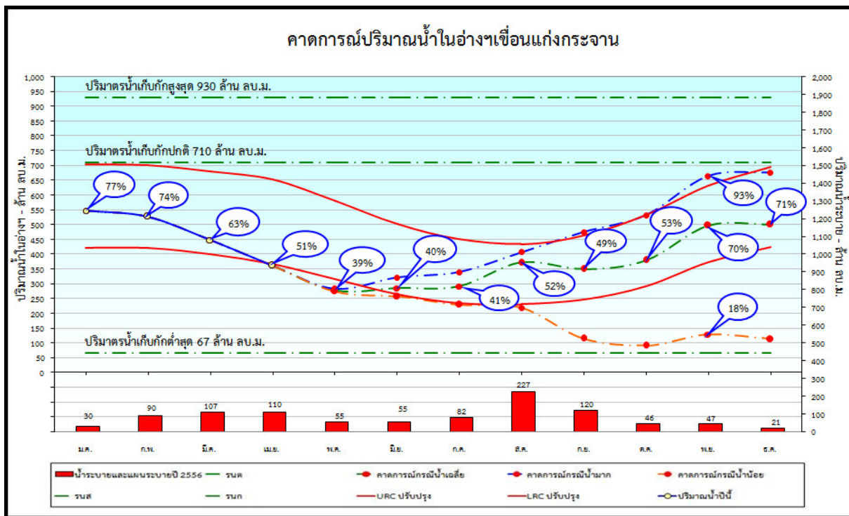
รูปที่ 30 การคาดการณ์ปริมาณน้ำเขื่อนแก่งกระจาน กรณีปีน้ำเฉลี่ย ของปี พ.ศ. 2556
