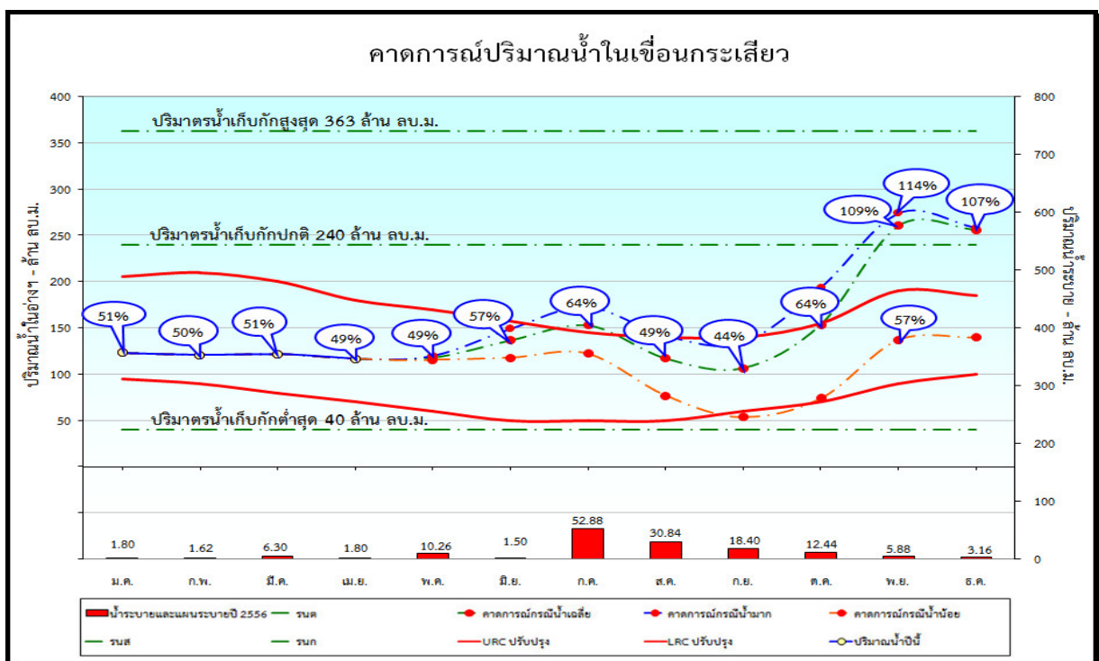
รูปที่ 22 การคาดการณ์ปริมาณน้ำเขื่อนกระเสียว กรณีปีน้ำเฉลี่ย ของปี พ.ศ. 2556
