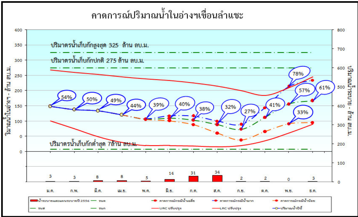
รูปที่ 17 การคาดการณ์ปริมาณน้ำเขื่อนลำแะะ กรณีปีน้ำเฉลี่ย ของปี พ.ศ. 2556
