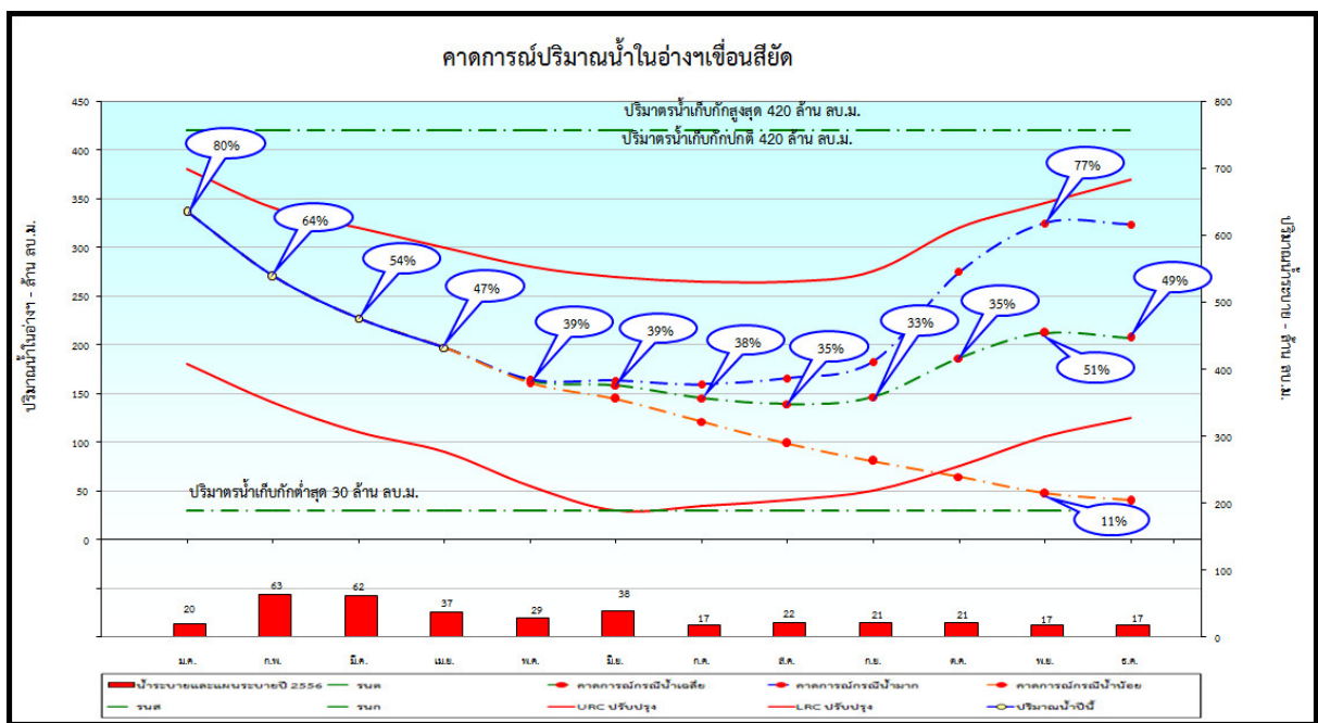
รูปที่ 26 การคาดการณ์ปริมาณน้ำเขื่อนสิียด กรณีปีน้ำเฉลี่ย ของปี พ.ศ. 2556
