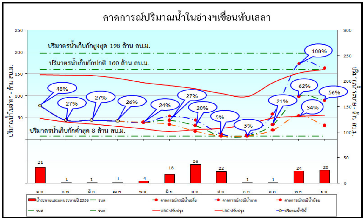
รูปที่ 21 การคาดการณ์ปริมาณน้ำเขื่อนทับเสลา กรณีปีน้ำเฉลี่ย ของปี พ.ศ. 2556
