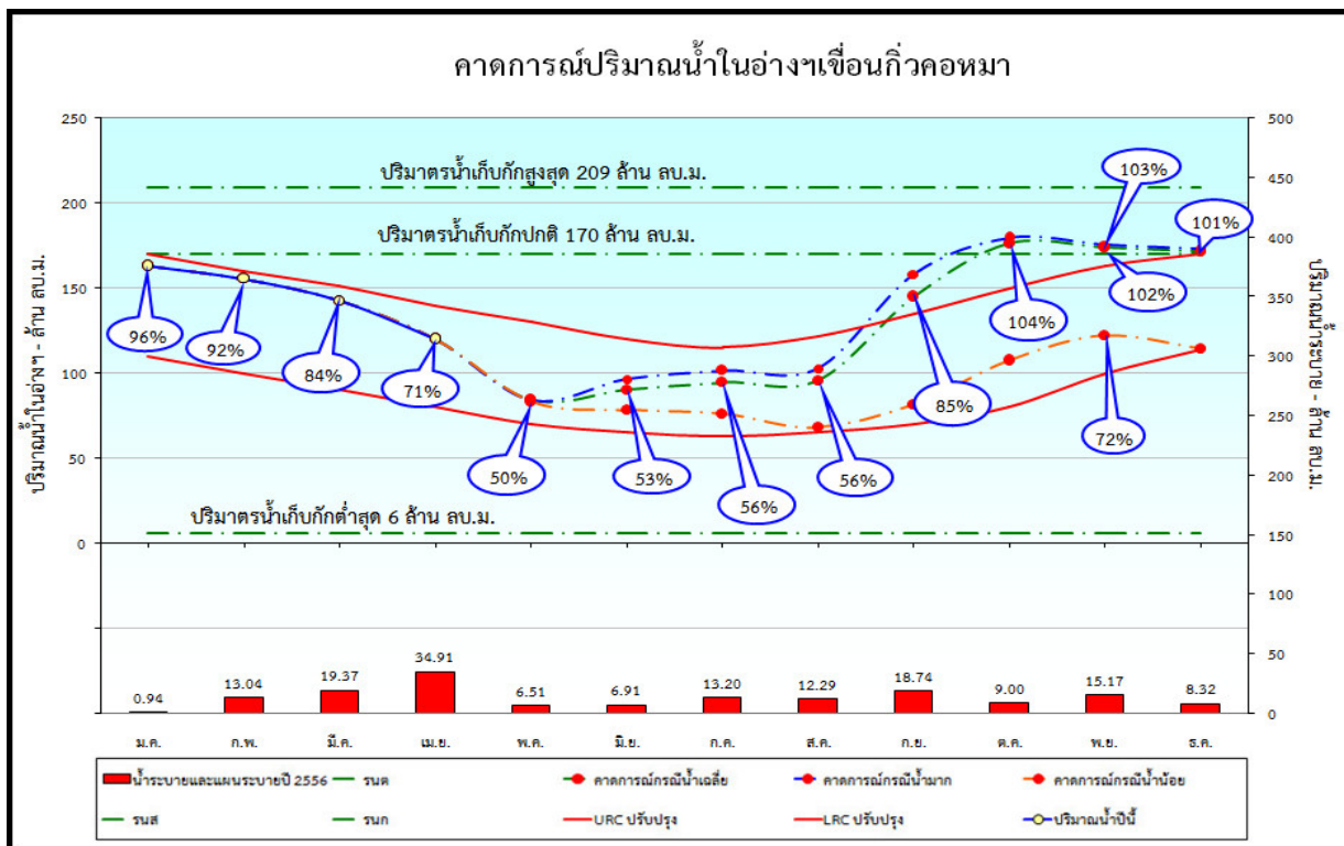
รูปที่ 6 การคาดการณ์ปริมาณน้ำเขื่อนกิ่วคอหมา กรณีปีน้ำเฉลี่ย ของปี พ.ศ. 2556
