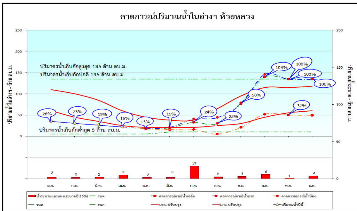
รูปที่ 8 การคาดการณ์ปริมาณน้ำเขื่อนห้วยหลวง กรณีปีน้ำเฉลี่ย ของปี พ.ศ. 2556
