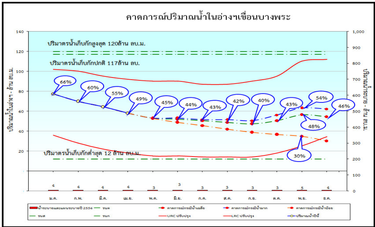
รูปที่ 27 การคาดการณ์ปริมาณน้ำเขื่อนบางพระ กรณีปีน้ำเฉลี่ย ของปี พ.ศ. 2556
