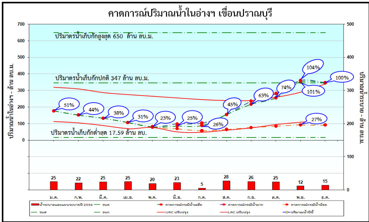
รูปที่ 31 การคาดการณ์ปริมาณน้ำเชื่อนปรามบุรี กรณีปีน้ำเฉลี่ย ของปี พ.ศ. 2556
