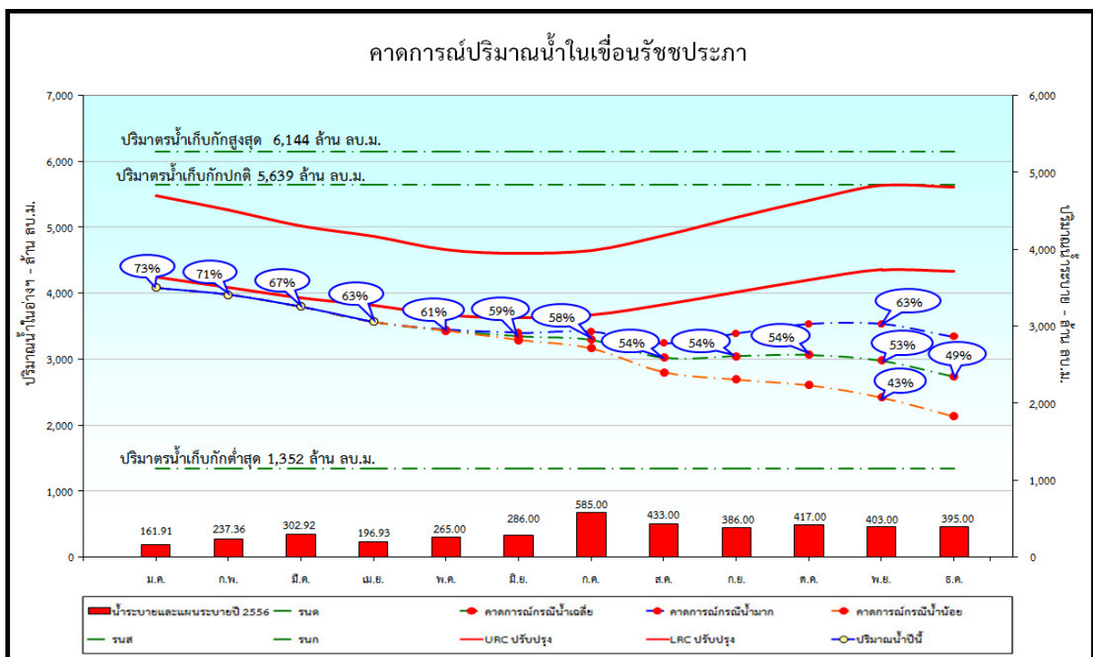
รูปที่ 32 การคาดการณ์ปริมาณน้ำเขื่อนรัชชประภา กรณีปีน้ำเฉลี่ย ของปี พ.ศ. 2556
