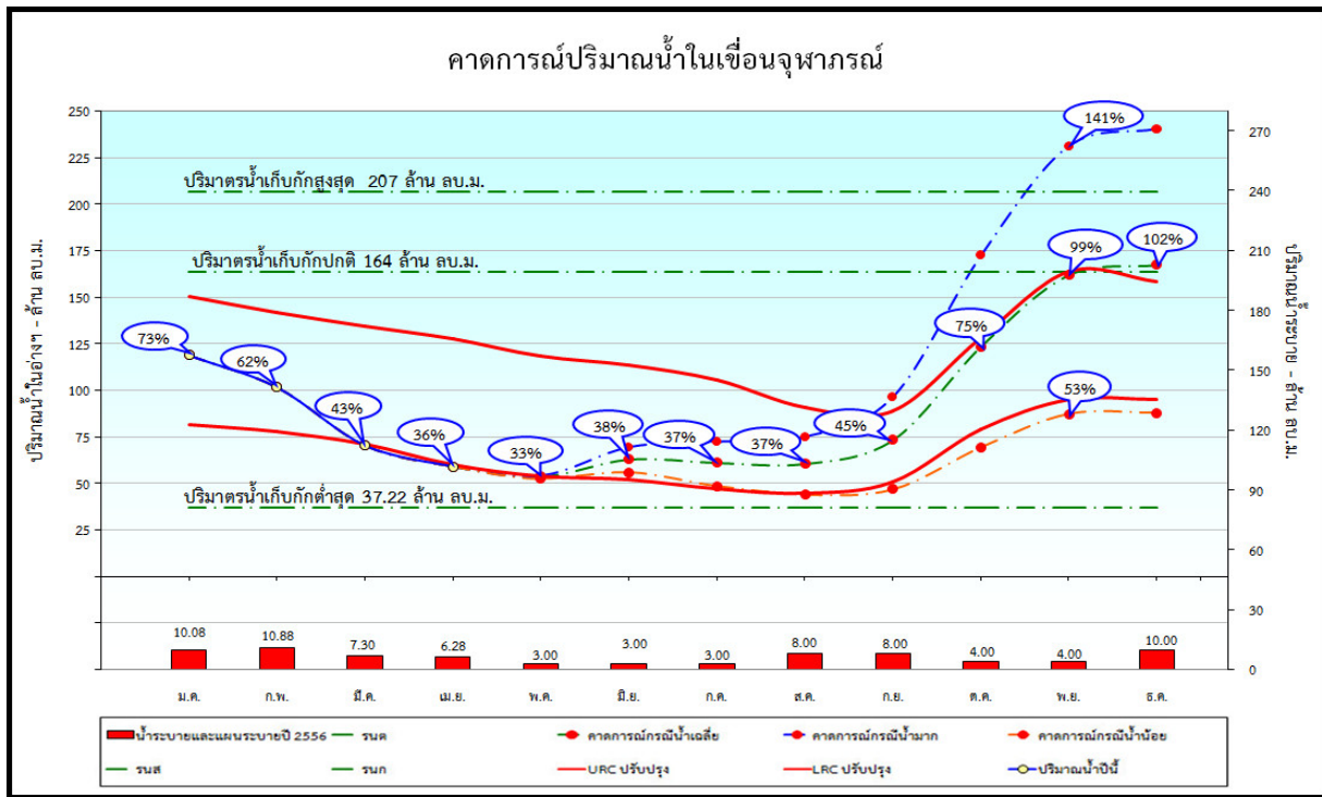
รูปที่ 11 การคาดการณ์ปริมาณน้ำเขื่อนจุฬาภรณ์ กรณีปีน้ำเฉลี่ย ของปี พ.ศ. 2556
