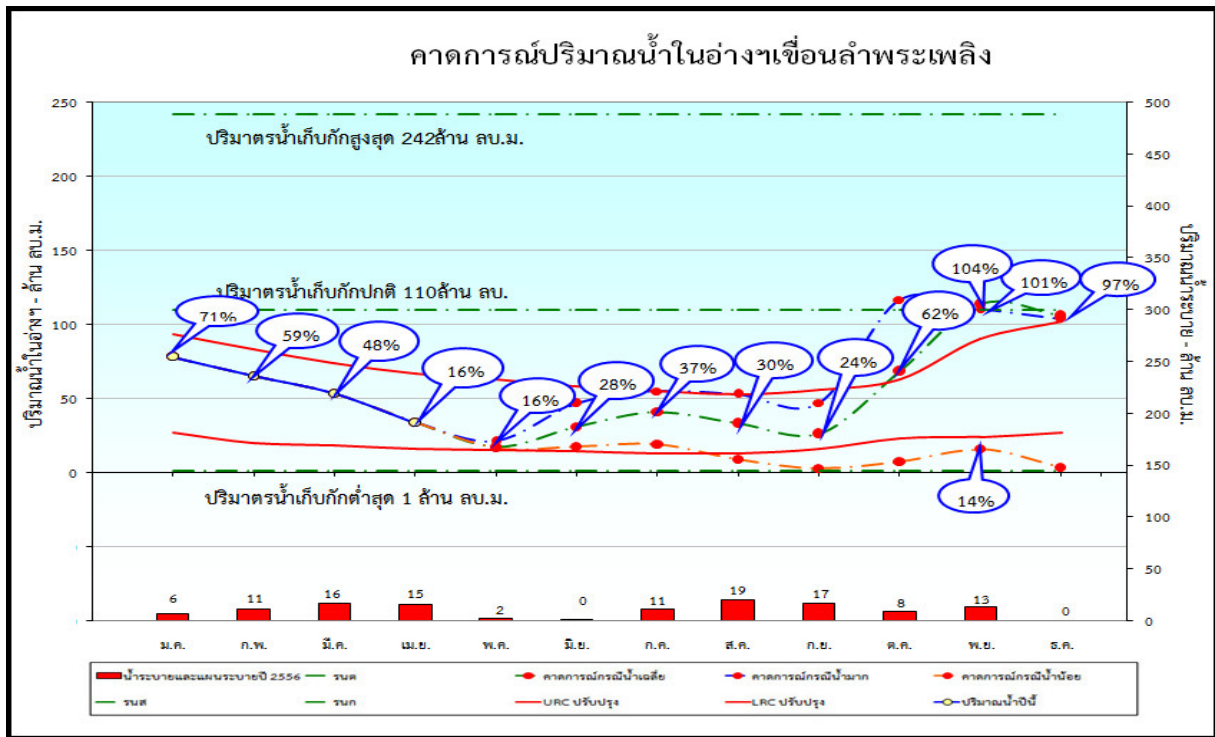
รูปที่ 15 การคาดการณ์ปริมาณน้ำเขื่อนลำพระเพลิง กรณีปีน้ำเฉลี่ย ของปี พ.ศ. 2556
