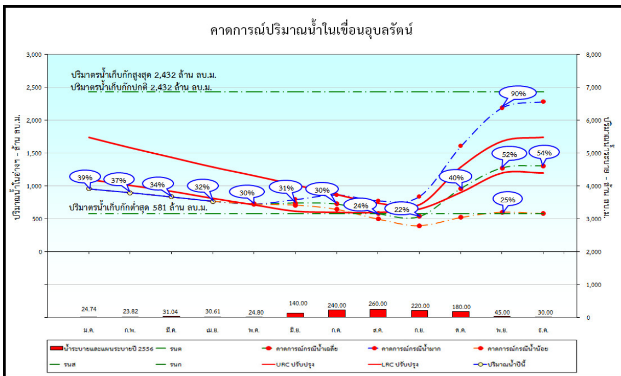
รูปที่ 12 การคาดการณ์ปริมาณน้ำเขื่อนอุบลรัตน์ กรณีปีน้ำเฉลี่ย ของปี พ.ศ. 2556
