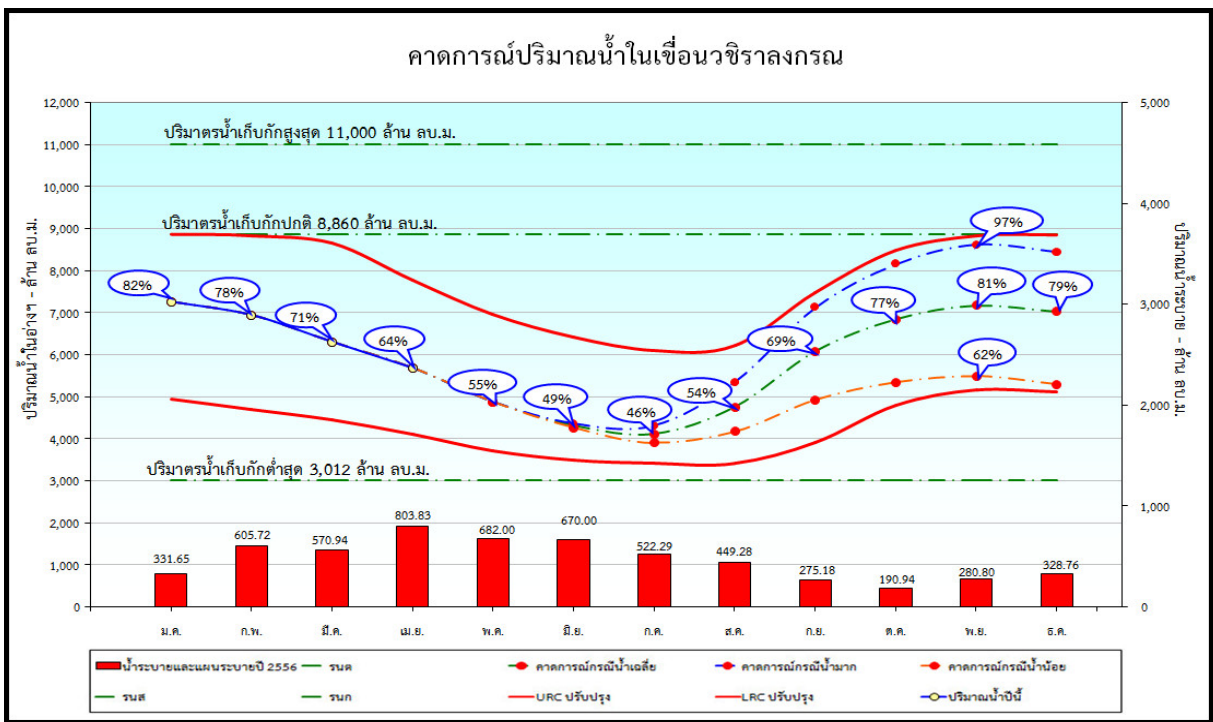
รูปที่ 24 การคาดการณ์ปริมาณน้ำเขื่อนวชิราลงกรณ กรณีปีน้ำเฉลี่ย ของปี พ.ศ. 2556
