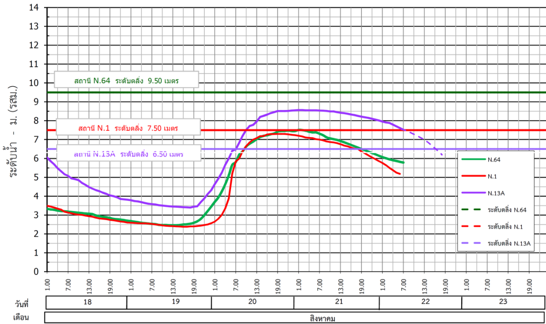
ระดับน้ำรายชั่วโมง ในลุ่มน้ำน่าน จ.น่าน
