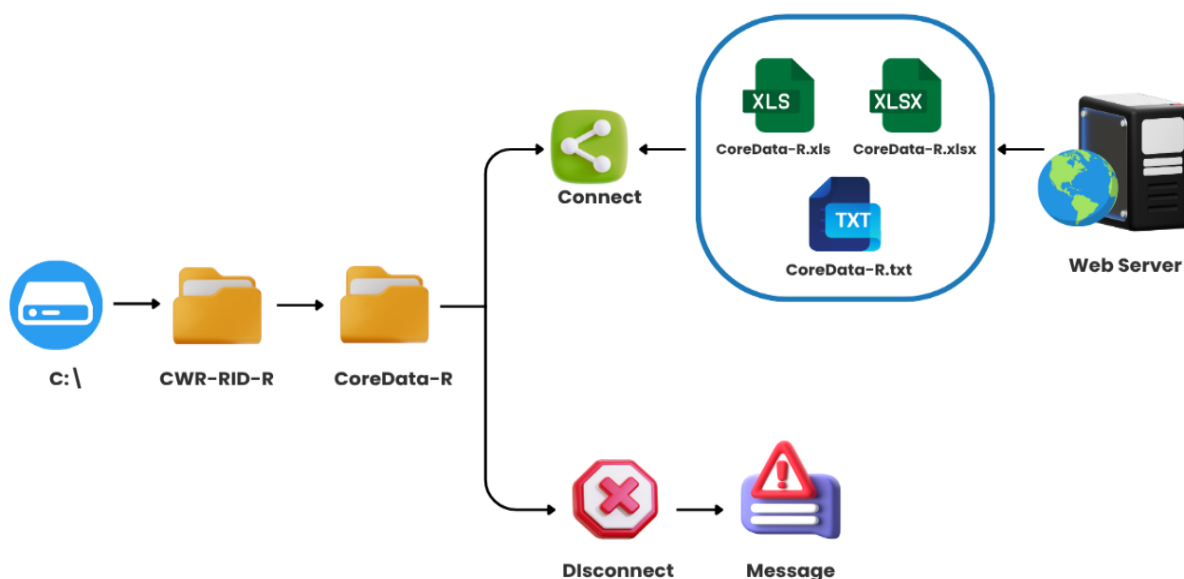
รูปที่ 7 ขั้นตอน Data Loading ... กรณีที่ไม่มีโฟลเดอร์ ไม่มีไฟล์ฐานข้อมูล หรือกรณีที่มีโฟลเดอร์ หรือมีไฟล์แต่มีไม่ครบ
