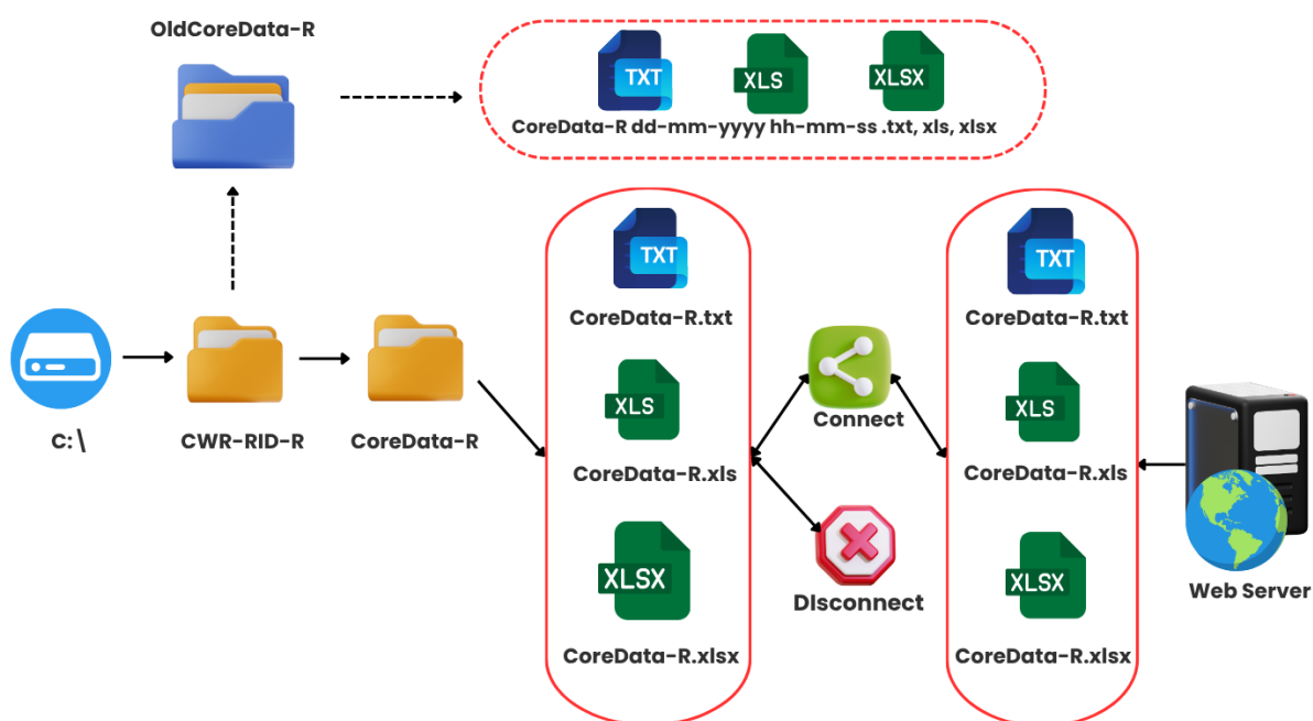
รูปที่ 8 ขั้นตอน Data Loading กรณีที่มีโฟลเดอร์ มีไฟล์ฐานข้อมูลครบ
